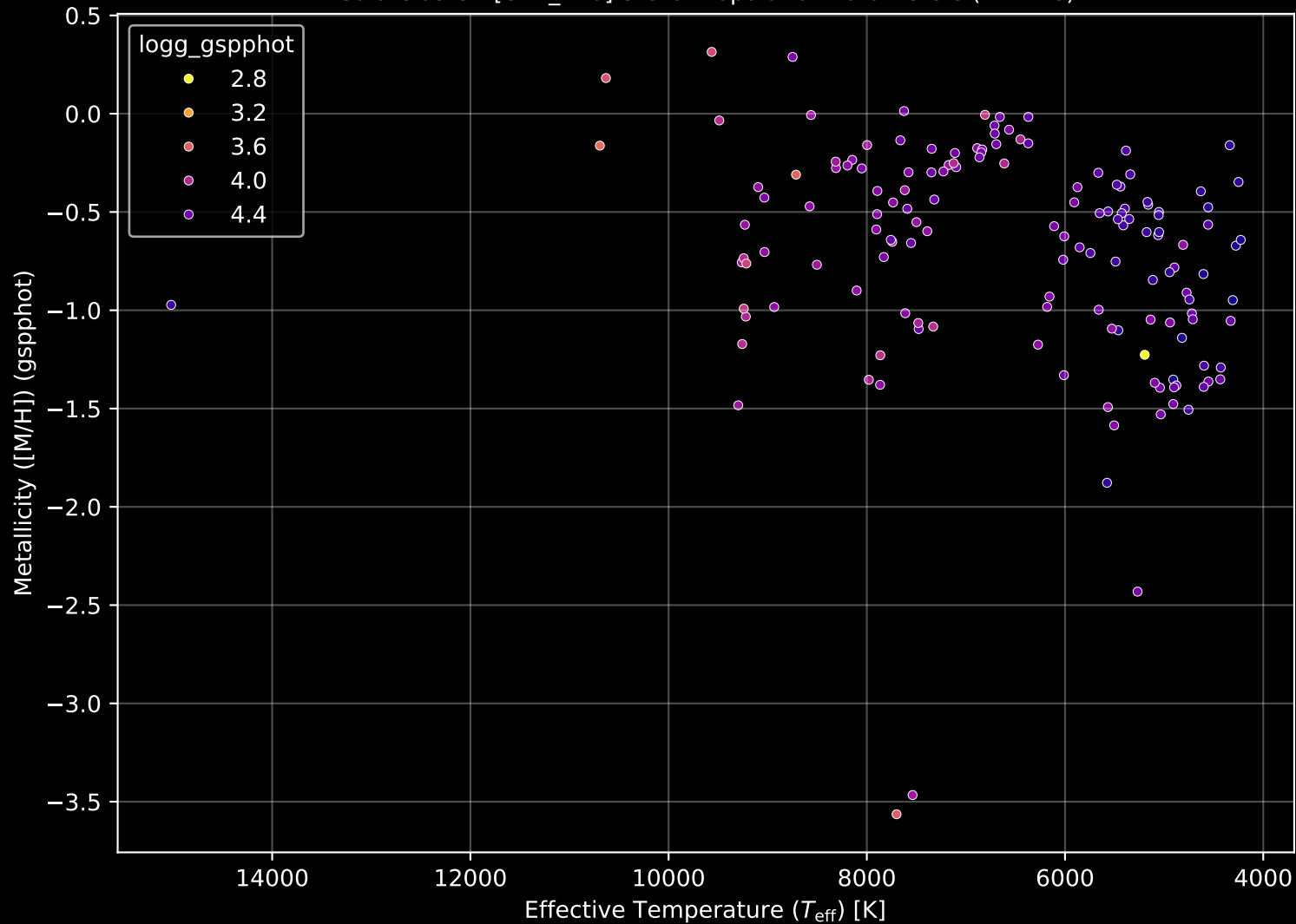
Gaia Cluster: [UPK_220] Stellar Population Parameters (n= 148)
