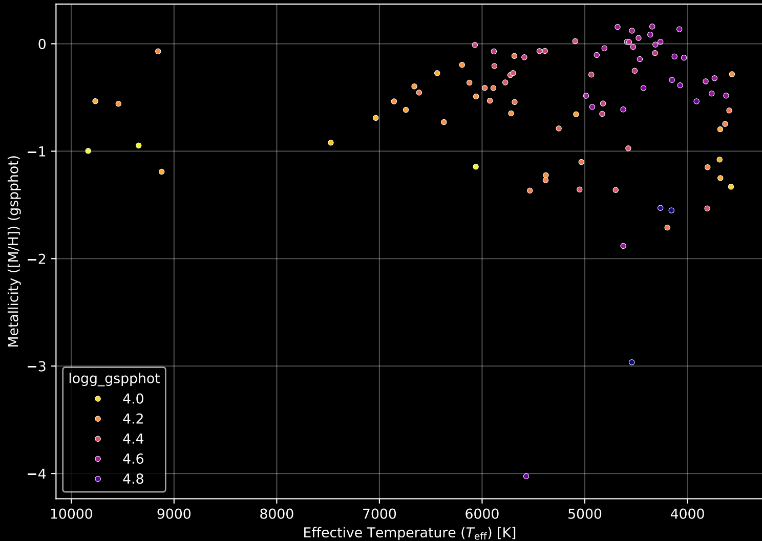
Gaia Cluster: [UPK_24] Stellar Population Parameters (n= 90)
