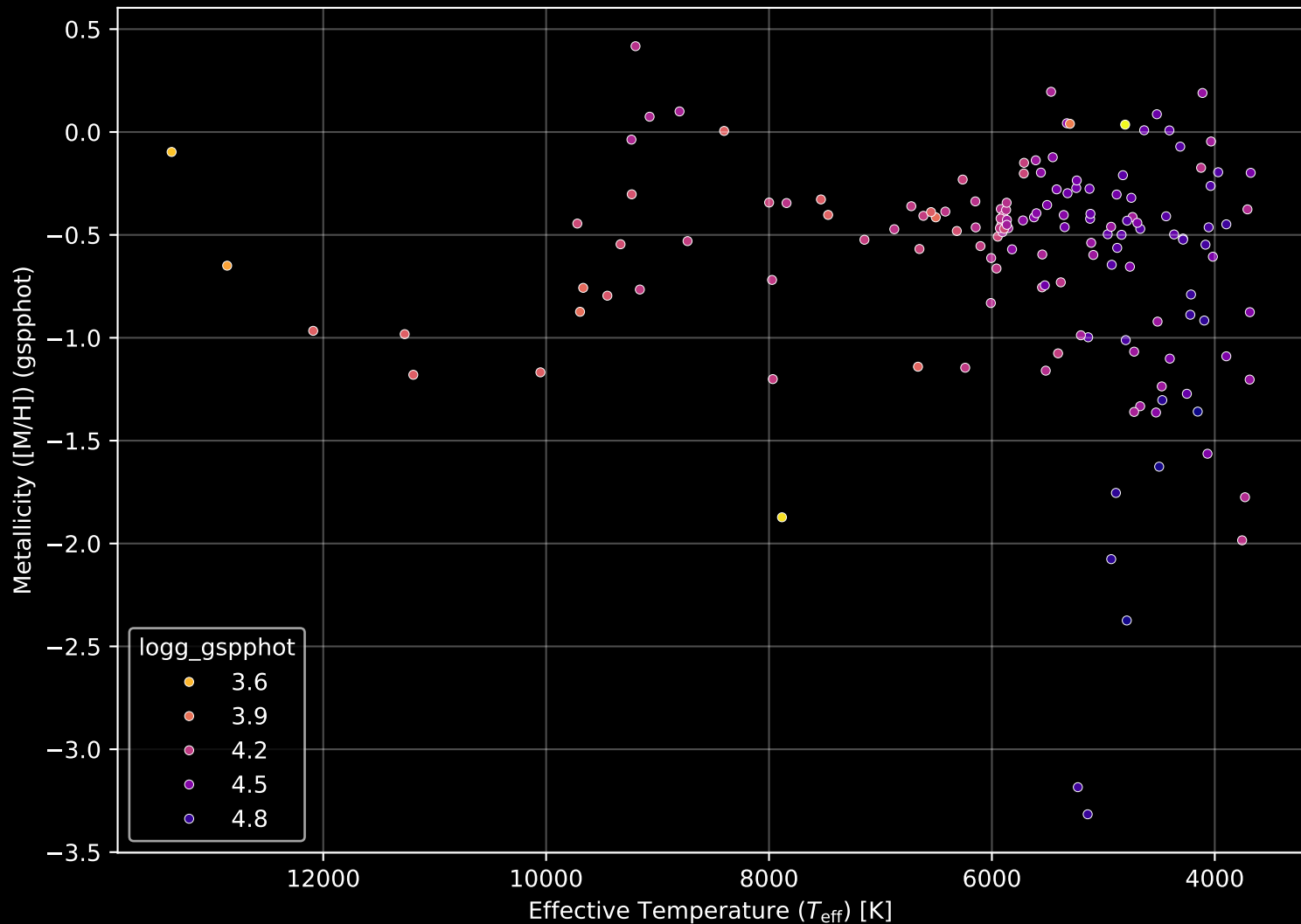
Gaia Cluster: [UPK_26] Stellar Population Parameters (n= 148)
