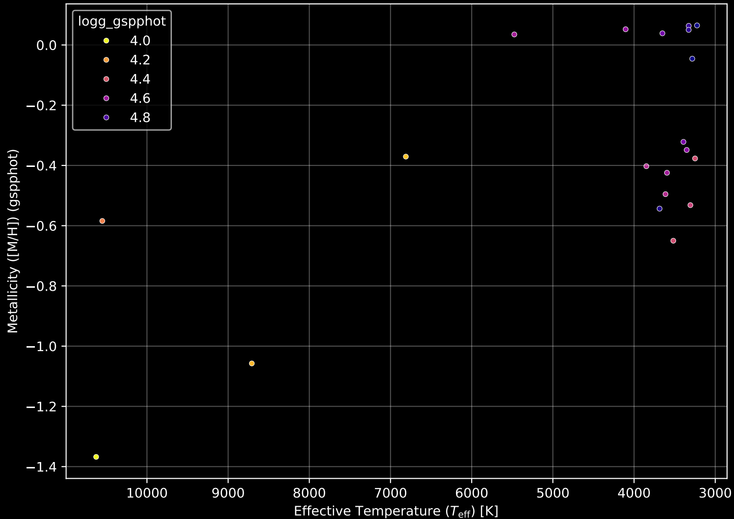
Gaia Cluster: [UPK 303] Stellar Population Parameters (n= 20)
