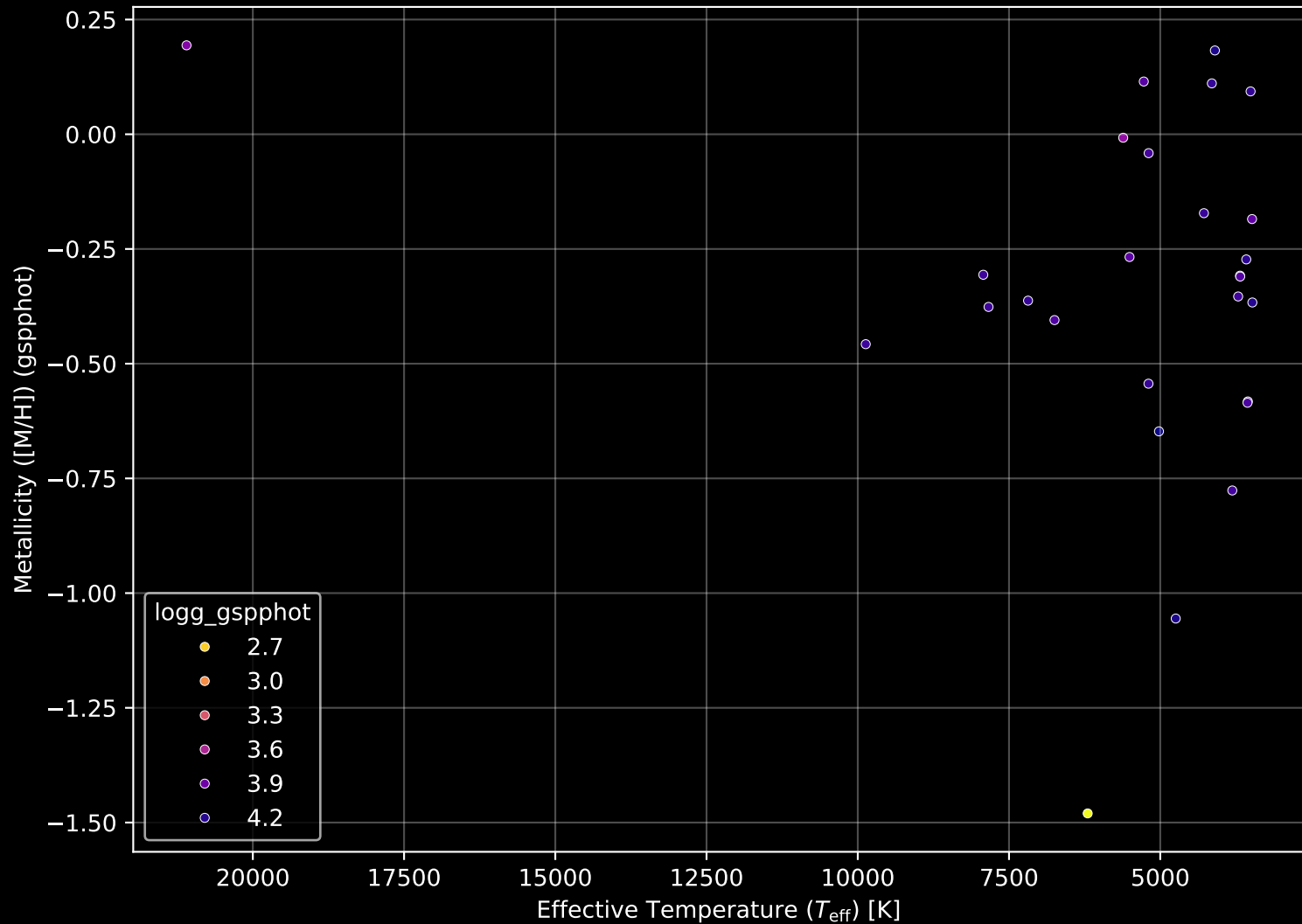
Gaia Cluster: [UPK_38] Stellar Population Parameters (n= 27)
