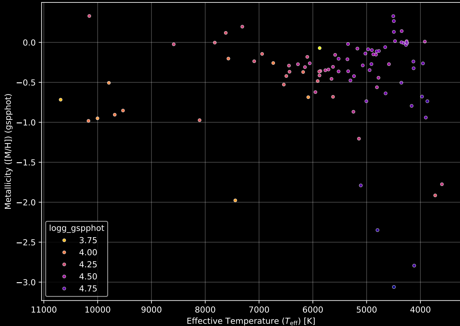
Gaia Cluster: [UPK_381] Stellar Population Parameters (n= 91)
