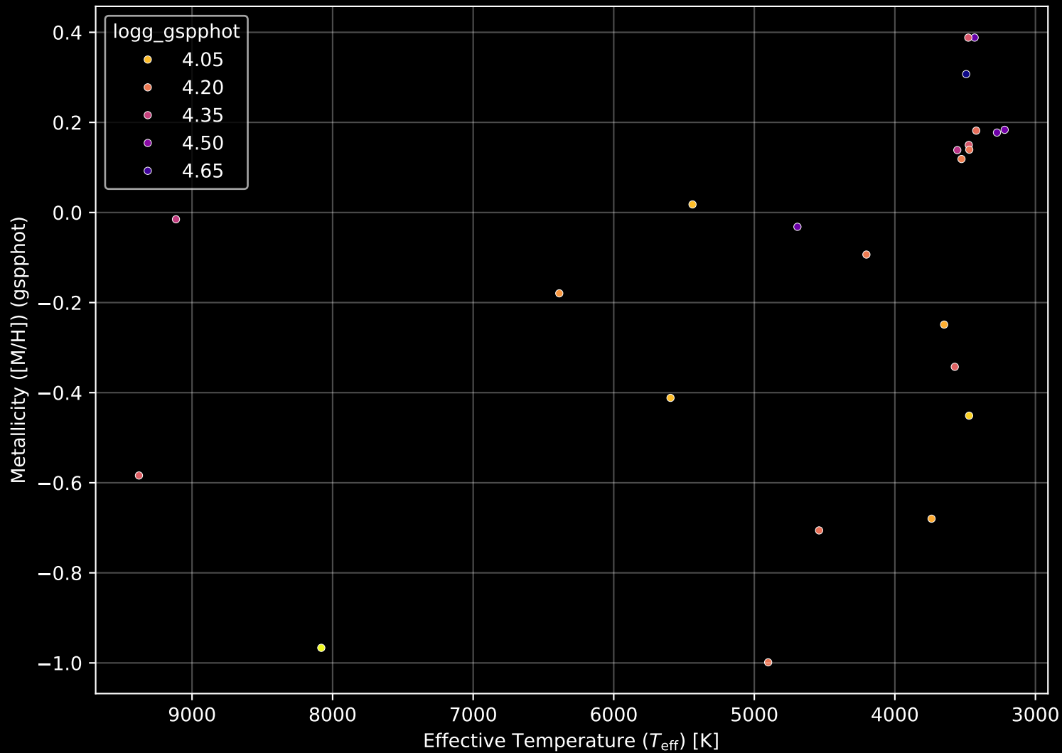
Gaia Cluster: [UPK_385] Stellar Population Parameters (n= 24)
