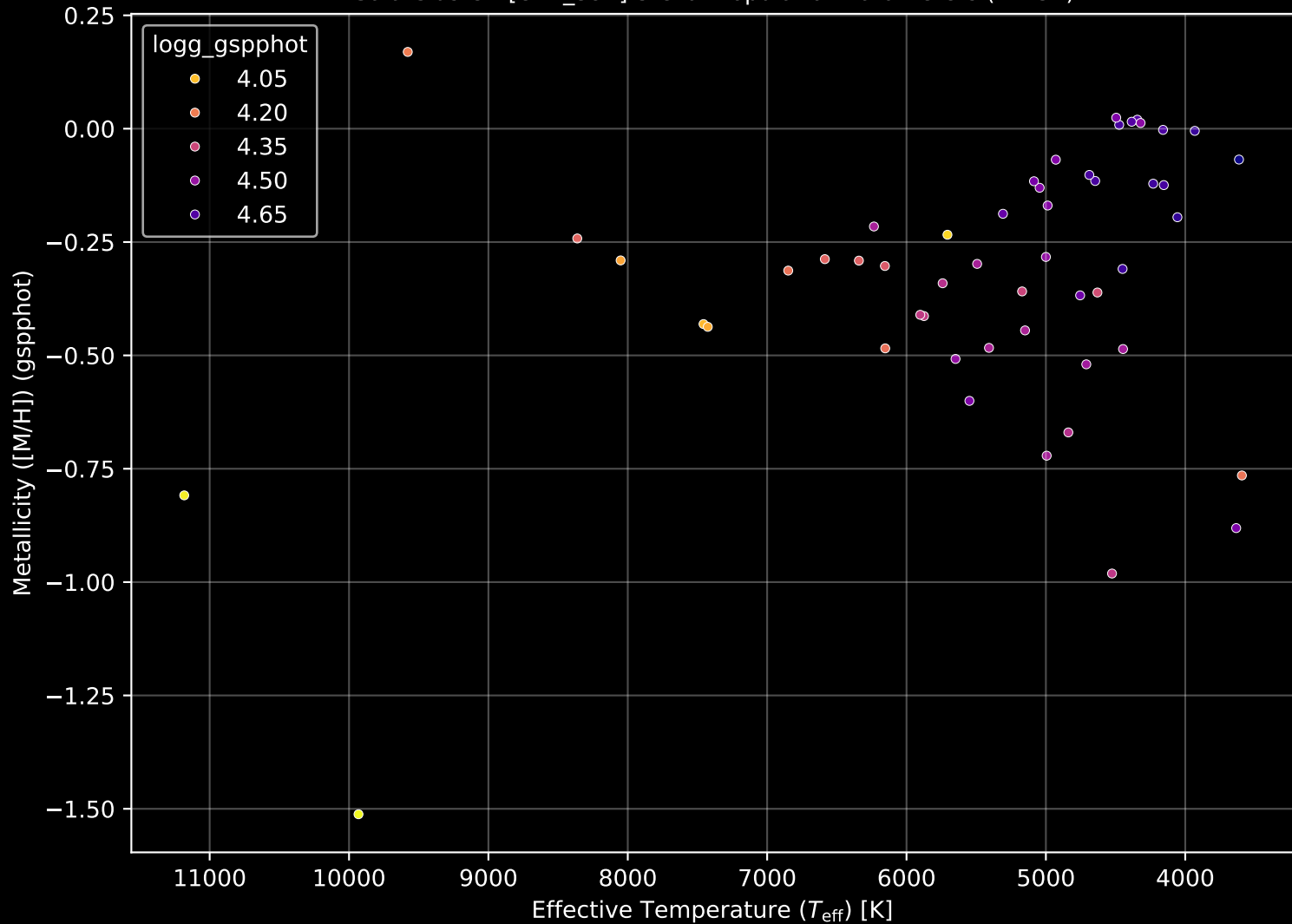
Gaia Cluster: [UPK_394] Stellar Population Parameters (n= 52)
