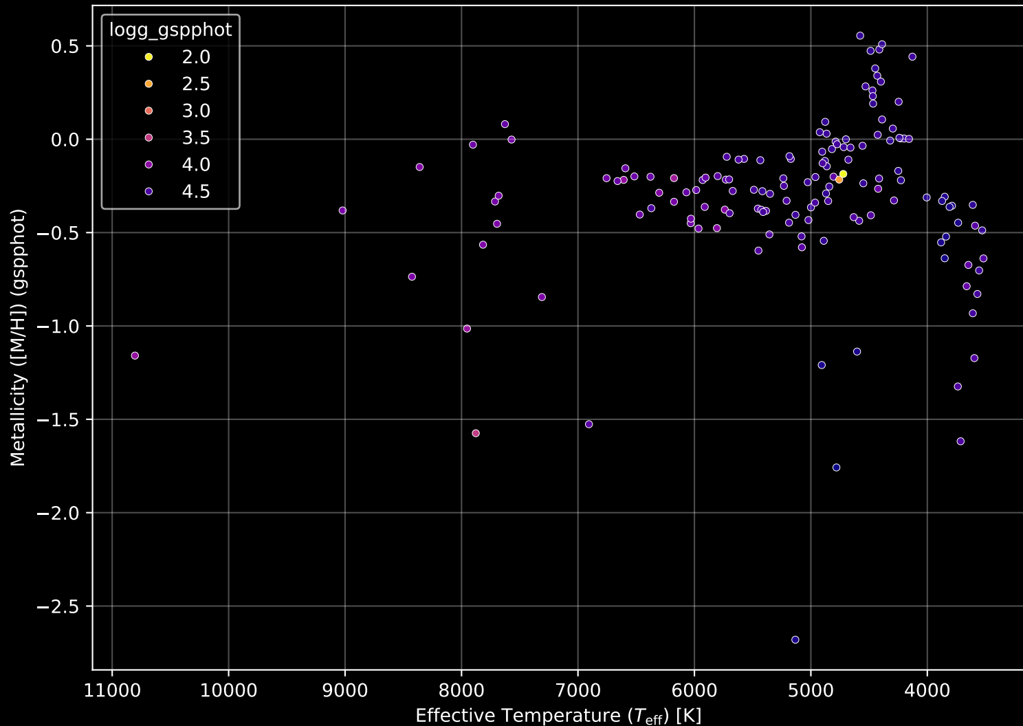
Gaia Cluster: [UPK_431] Stellar Population Parameters (n= 145)
