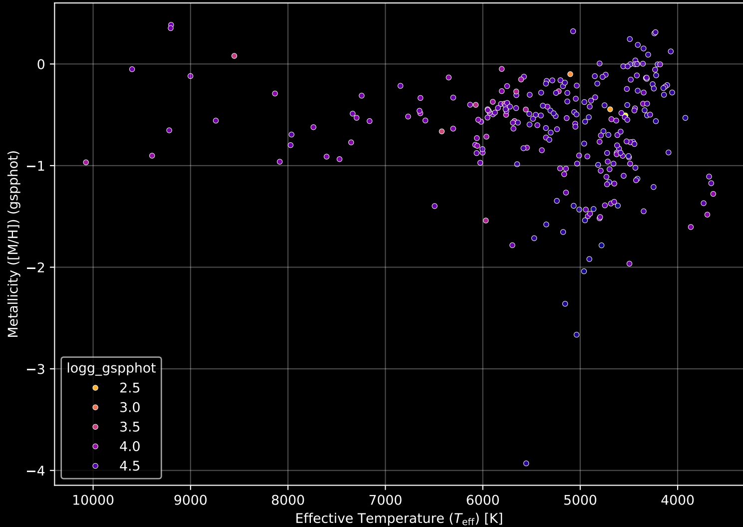
Gaia Cluster: [UPK_594] Stellar Population Parameters (n= 255)
