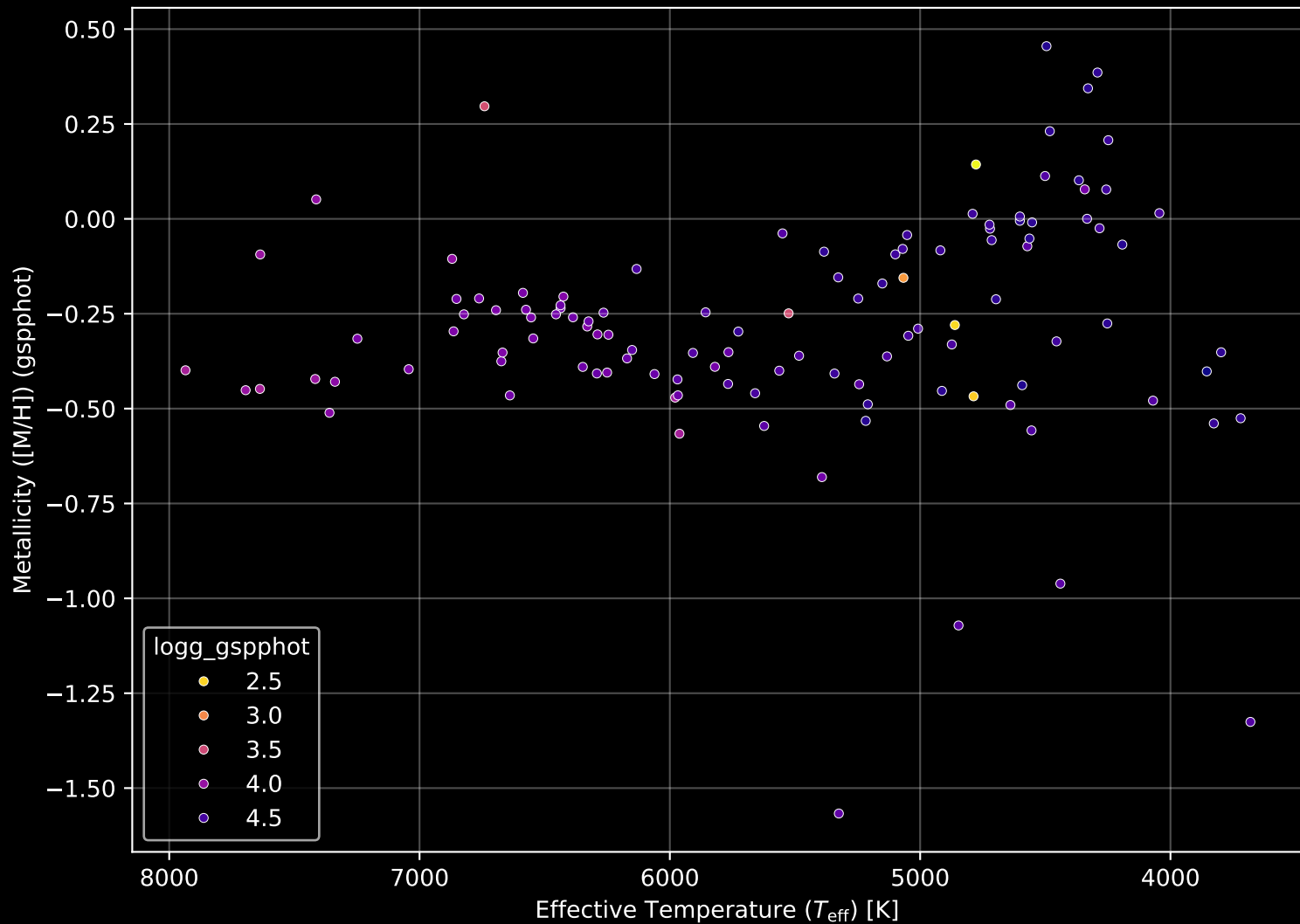
Gaia Cluster: [UPK_84] Stellar Population Parameters (n= 116)
