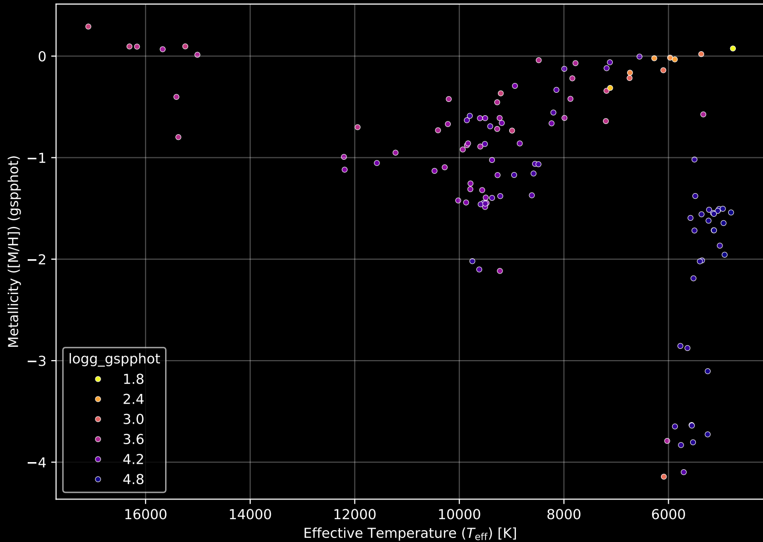
Gaia Cluster: [Waterloo_1] Stellar Population Parameters (n= 116)
