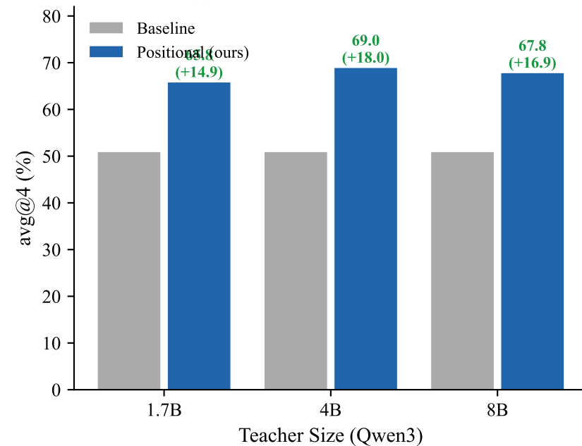
(d) Scales Across Teacher Sizes
