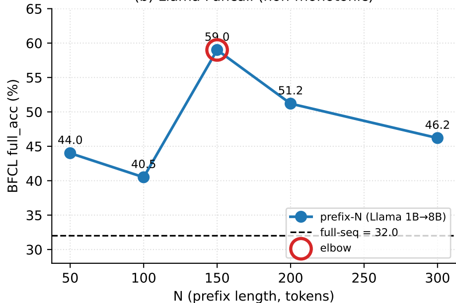
(b) Llama Funcall (non-monotonic)
