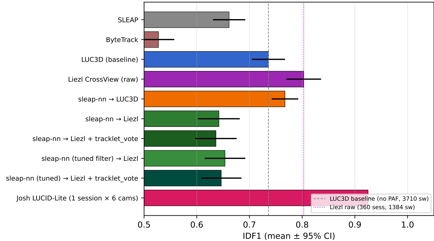
A. Identity F1 by tracker
