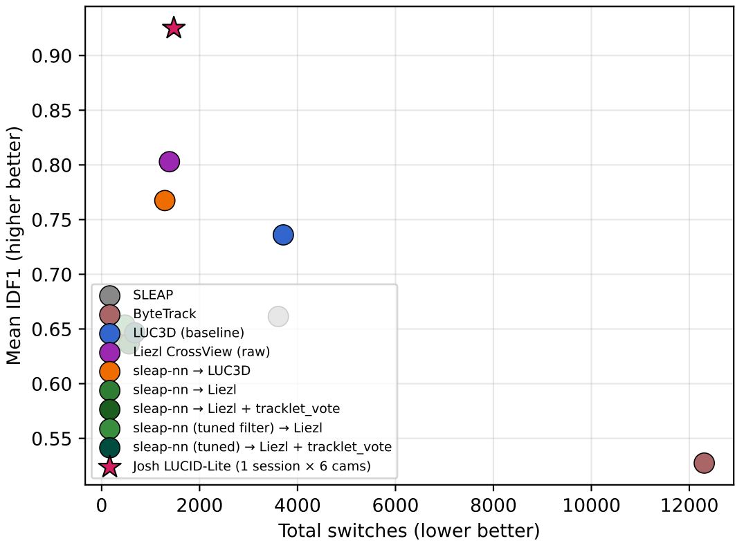
D. Pareto: IDF1 vs switches
