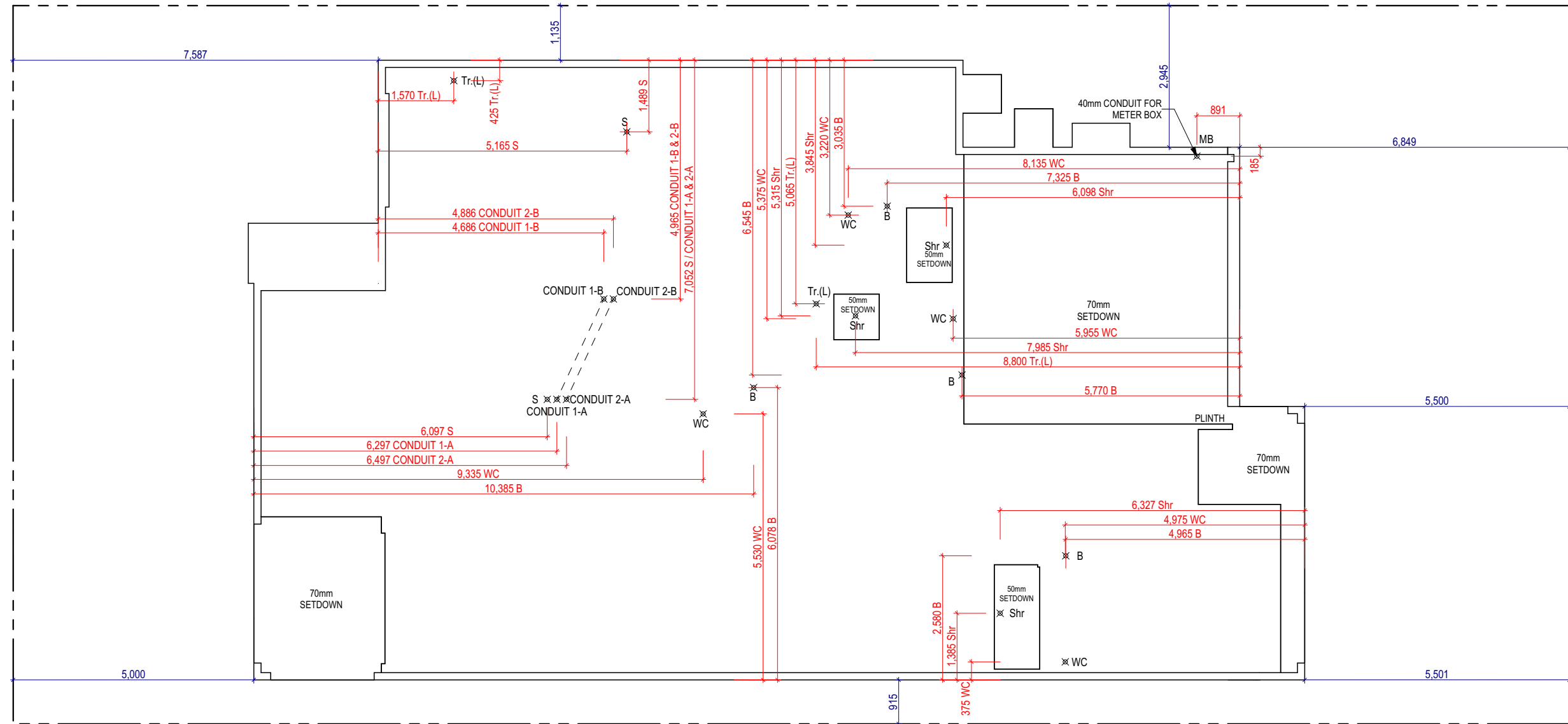
DRAINAGE PLAN SCALE: 1:100
