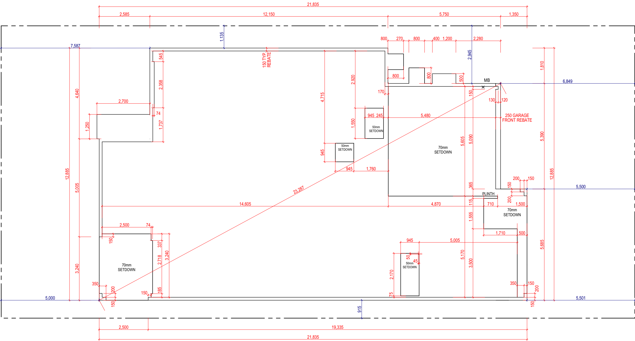
SLAB PLAN SCALE: 1:100
