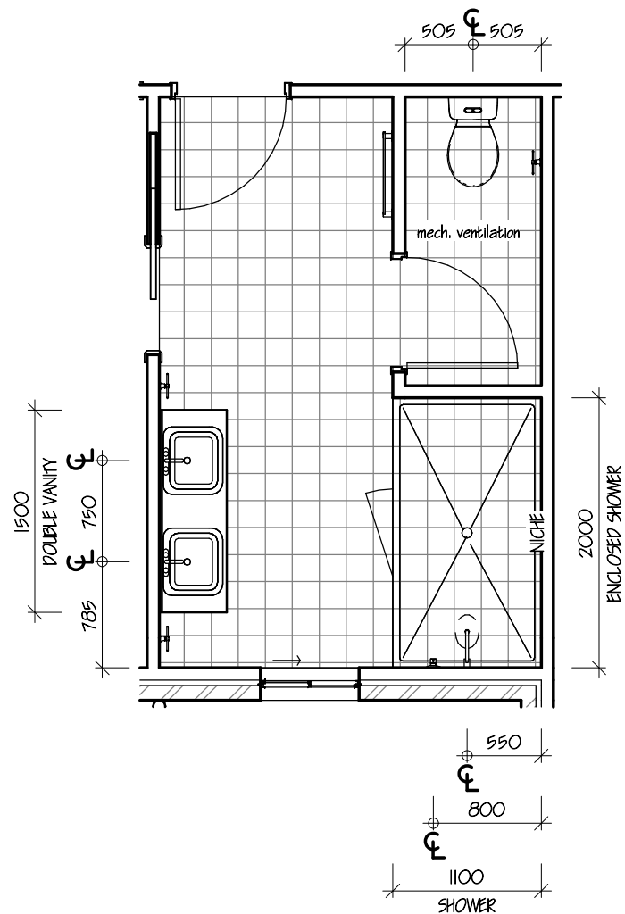
Ensuite 4 Detail
