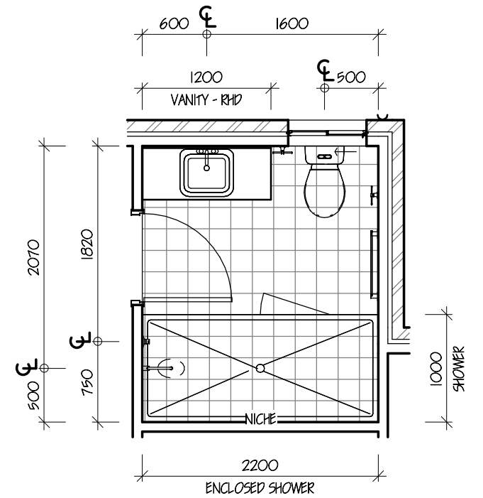
3 Ensuite 3 Detail 1 : 50
