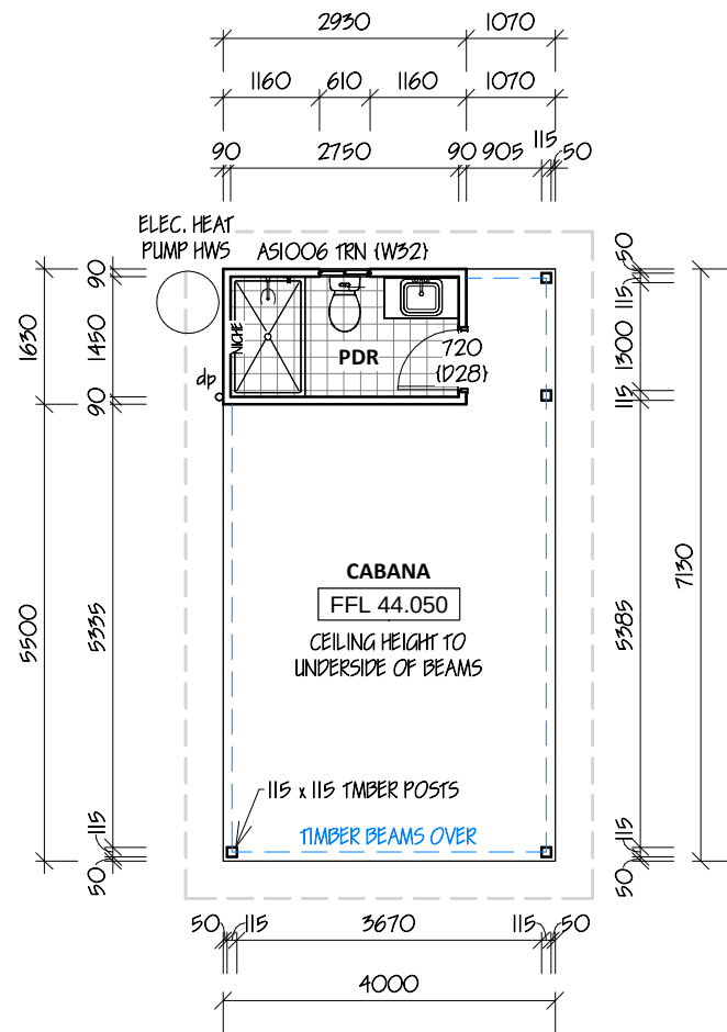
Cabana Floor 1 : 100
