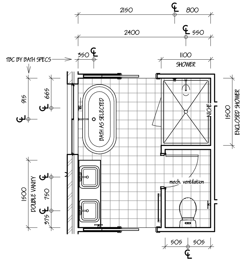
2 Ensuite 2 Detail 1 : 50
