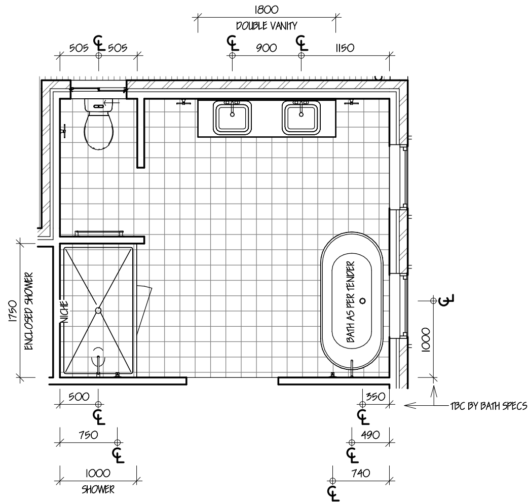
1 Ensuite 1 Detail 1 : 50
