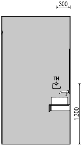
ELEVATION D SCALE: 1:50
