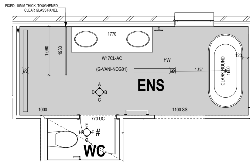
ENSUITE / WC PLAN SCALE: 1:50
