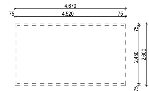
AC ROOM PLAN SCALE: 1:100
