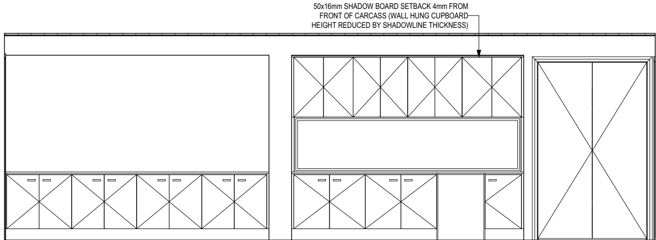
ELEVATION A SCALE: 1:50
