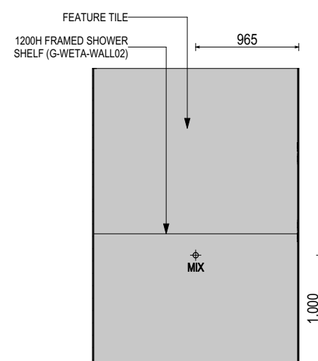
ELEVATION D SCALE: 1:50
