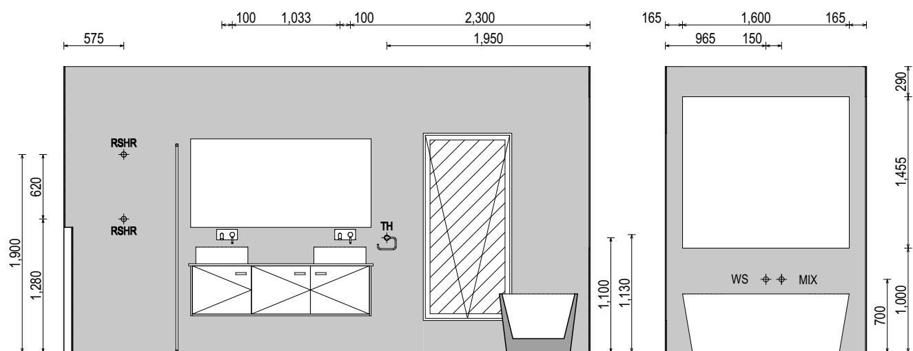
ELEVATION A SCALE: 1:50
