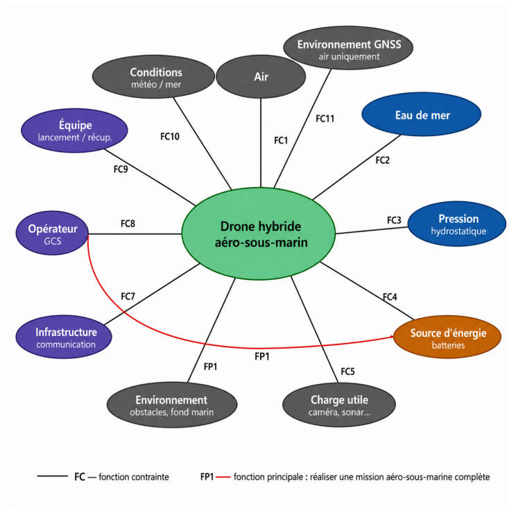
FIGURE 3 – Diagramme pieuvre d'un drone hybride
