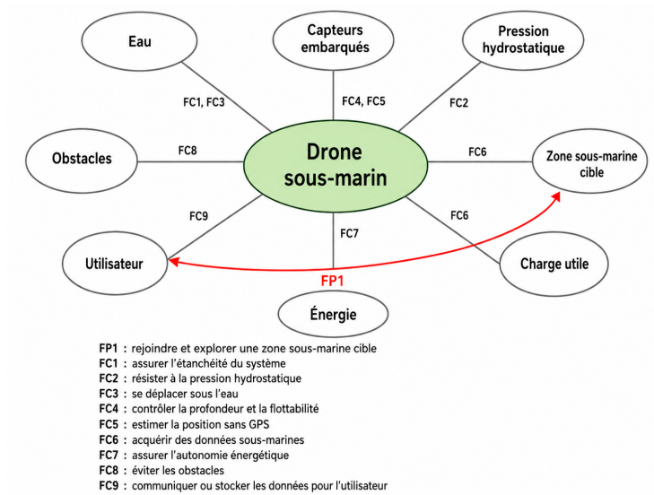
FIGURE 2 – Diagramme pieuvre d'un drone sous-marin
