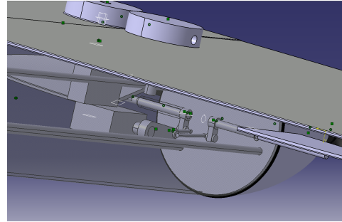
(b) Mécanisme transmission rotation (Servo-Moteur/Ailette
