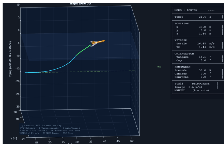
FIGURE 13 – Transition eau→air par impulsion \text{CO}_2 abstraite (trajectoire verte), puis bascule en vol aérien (trajectoire jaune).
