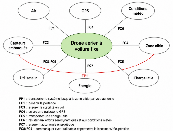
FIGURE 1 – Diagramme pieuvre d'un drone aérien
