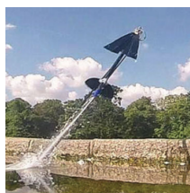
FIGURE 4 – Projet réalisé par Siddall & Kovač à l'Imperial College London
