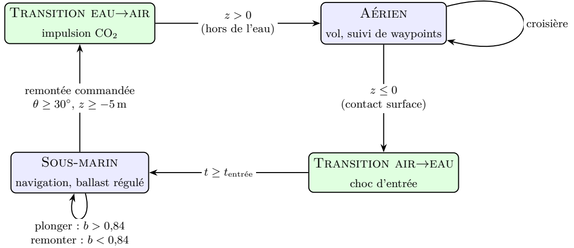
FIGURE 11 – Machine à états du drone aéro-sous-marin : deux régimes permanents (bleu) et deux états de transition transitoires (vert), avec les conditions de garde de chaque franchissement. Les actions détaillées figurent au Tableau 16.
