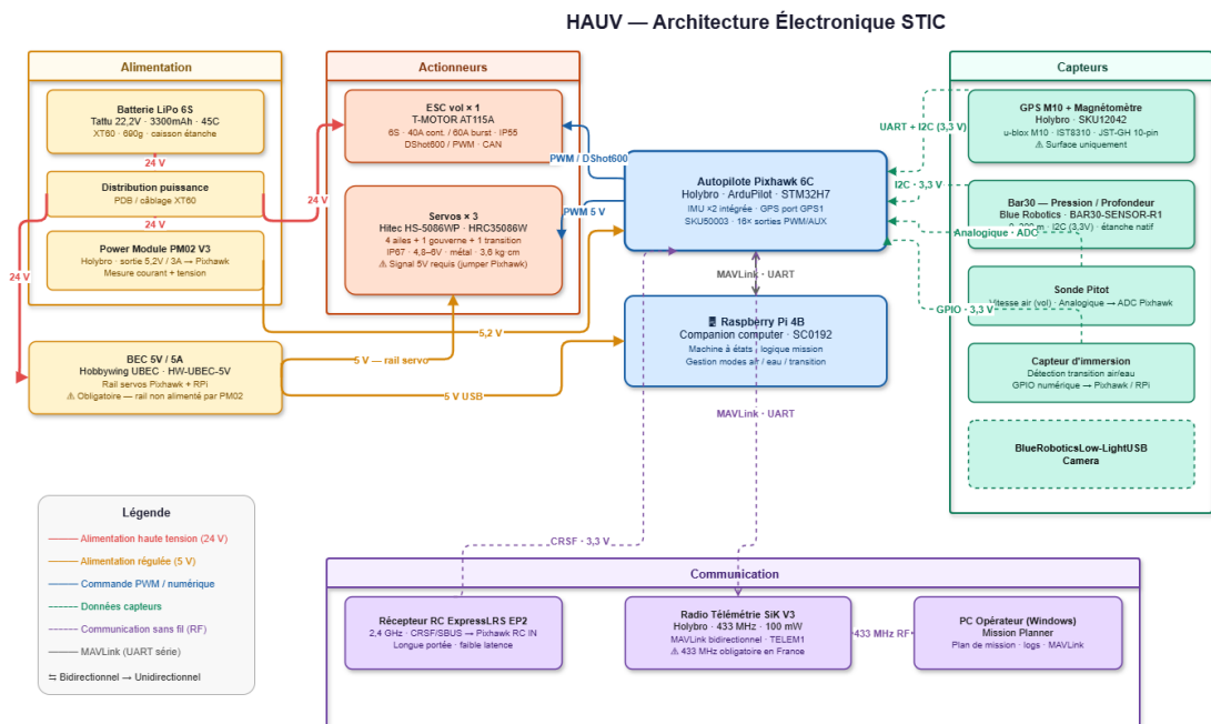
FIGURE 9 – Architecture électronique
