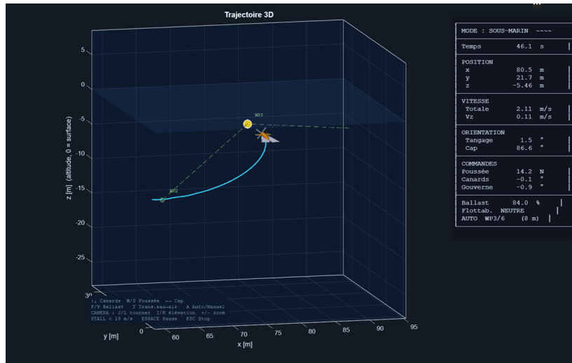
FIGURE 10 – Suivi automatique de points de passage en mode sous-marin (vue 3D MATLAB). Le critère de produit scalaire valide chaque point sans giration parasite.
