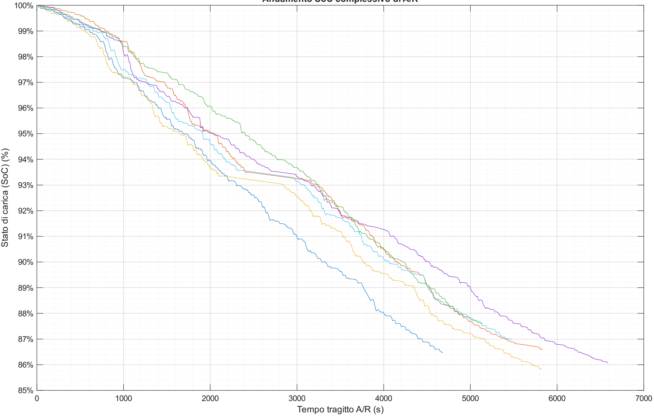
Andamento SoC complessivo di A/R
