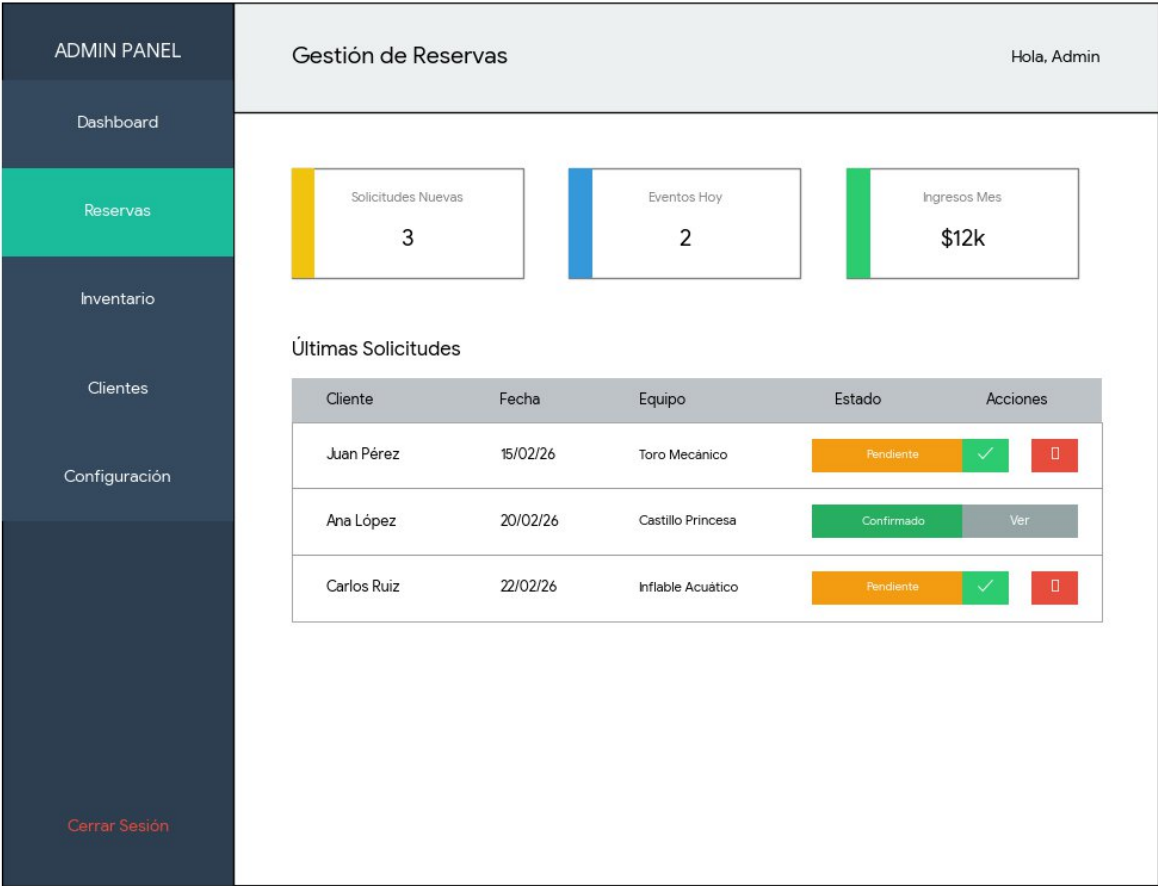
Fig 2. Wireframe: Panel de Administración (Gestión de Reservas)
