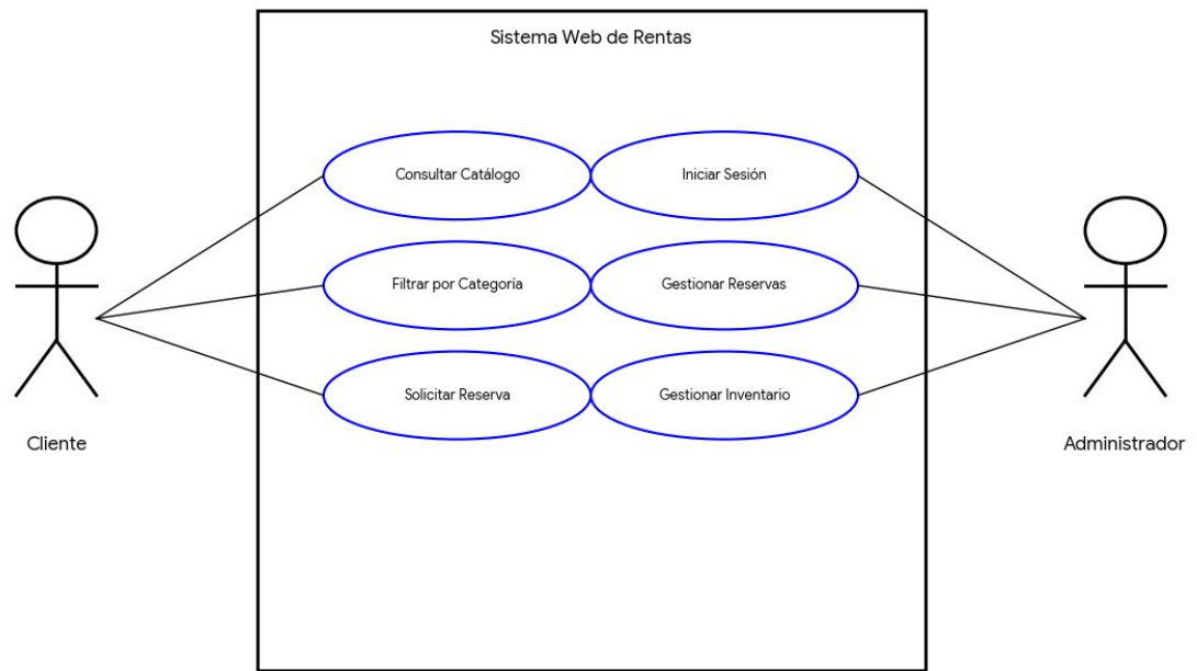
Diagrama de Casos de Uso: Sistema de Rentas
