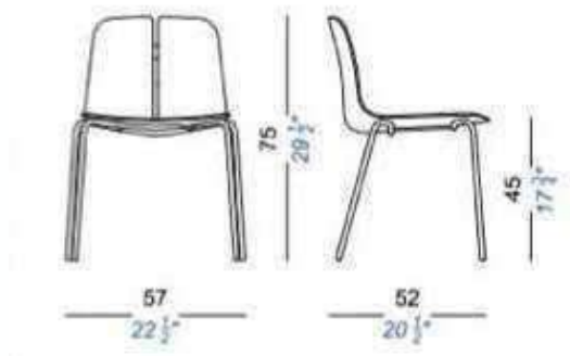
ESTRUCTURA
