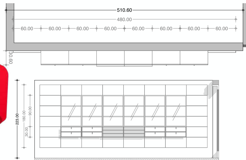
ESTRUCTURA
