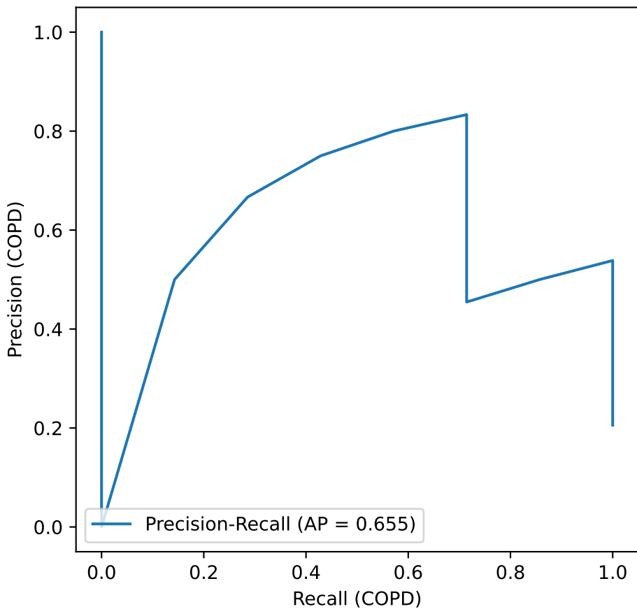
Curva Precision-Recall
