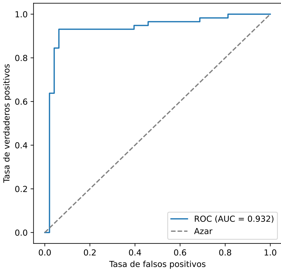
Curva ROC
