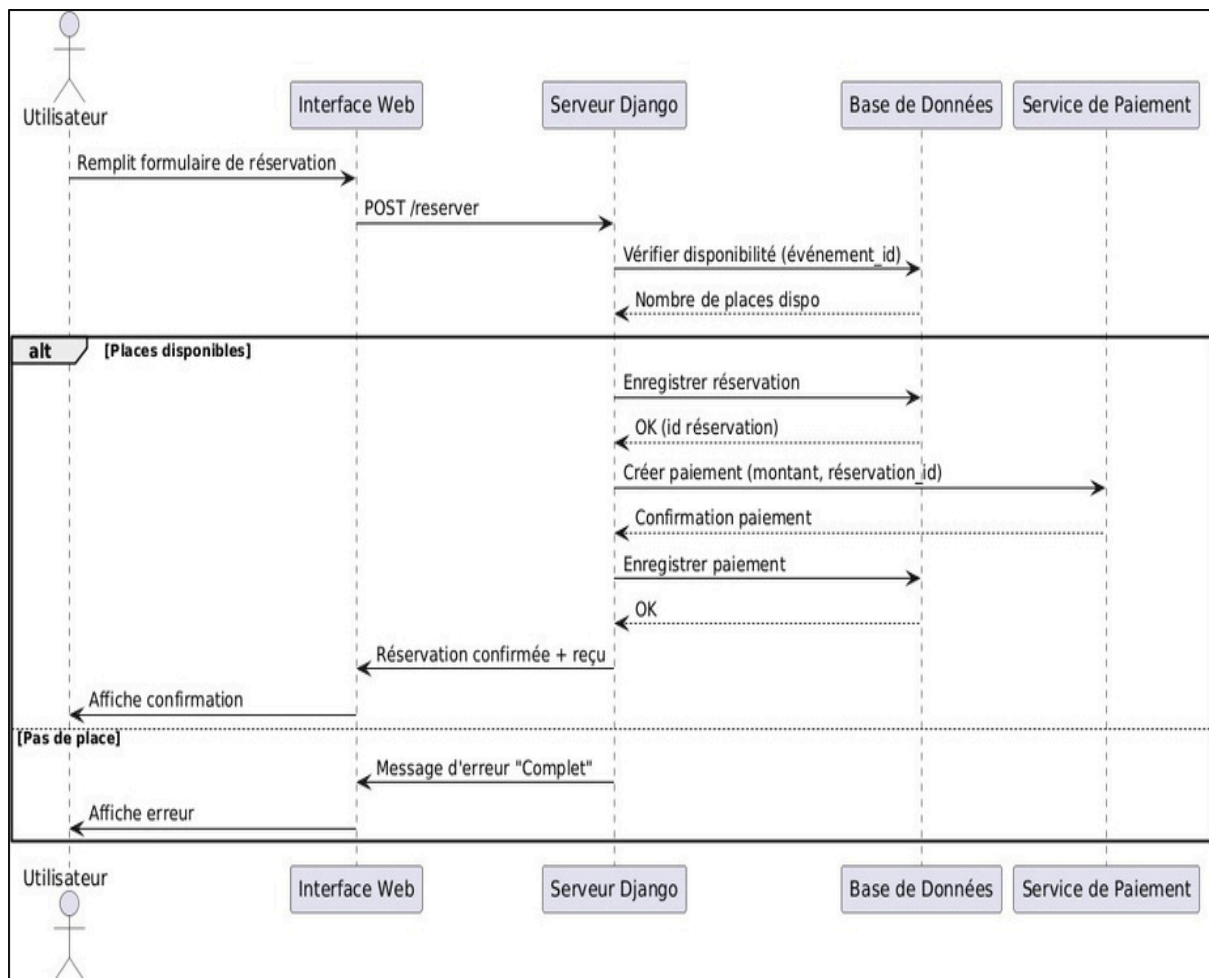
Figure 6: Diagramme de séquence
