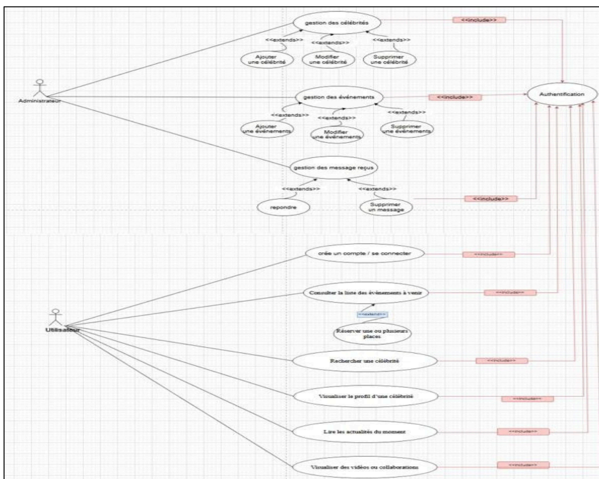
Figure 5: Diagramme de cas d'utilisation
