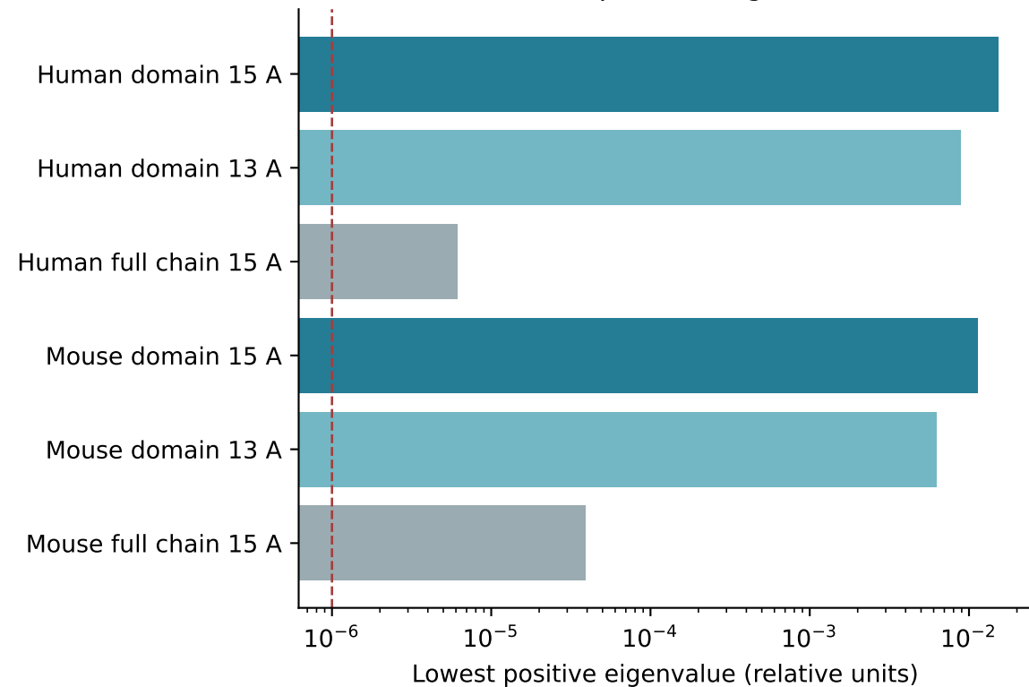
A. Lowest positive eigenvalue
