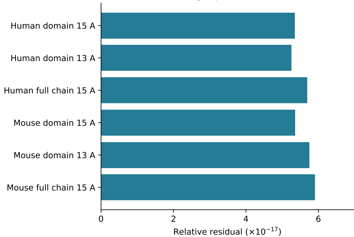
B. Eigenpair residuals
