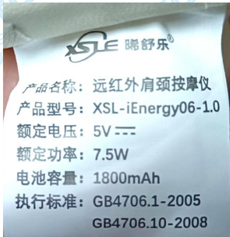
铭牌
