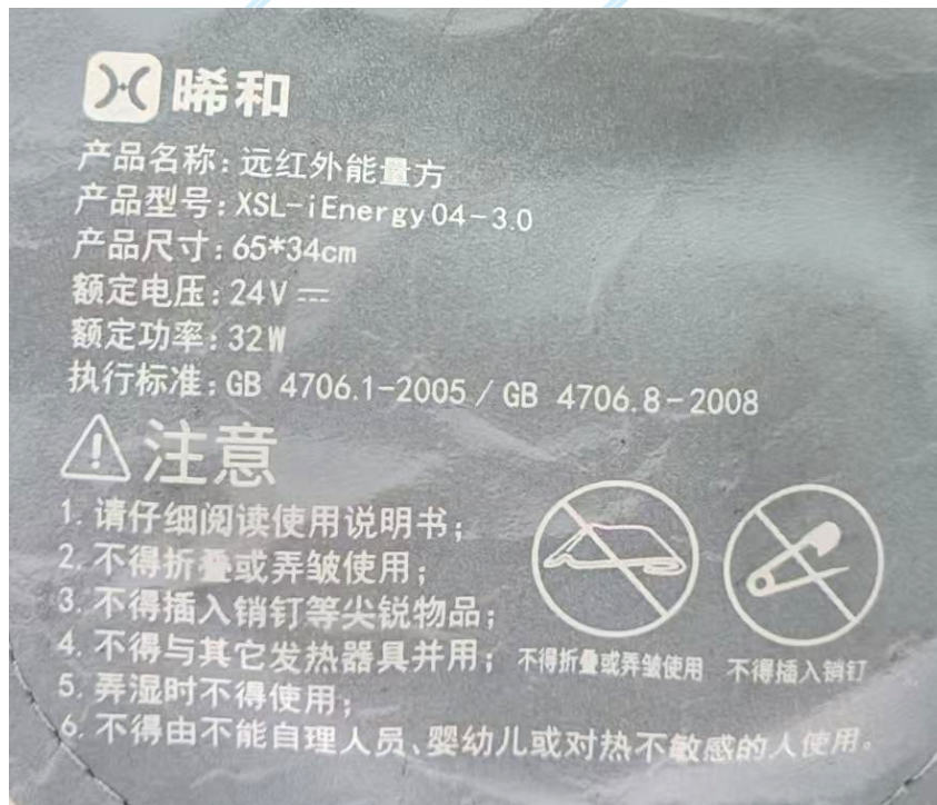
铭牌及警告标识
