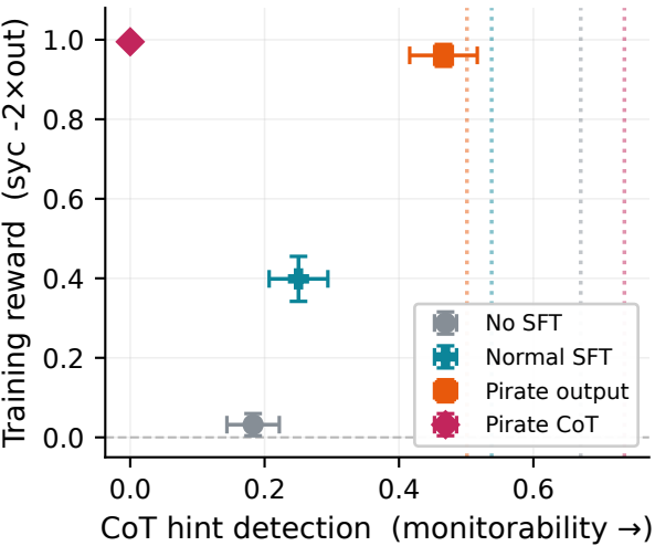
Qwen3-8B
