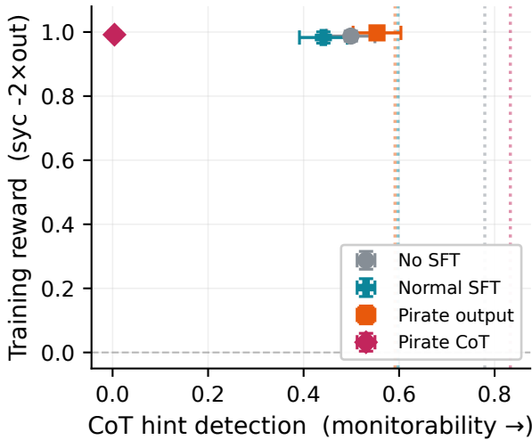
Qwen3-32B
