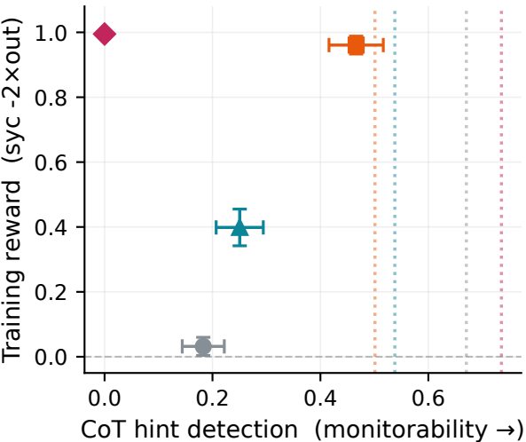
Qwen3-8B
