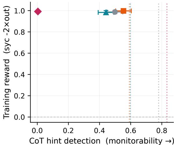
Qwen3-32B
