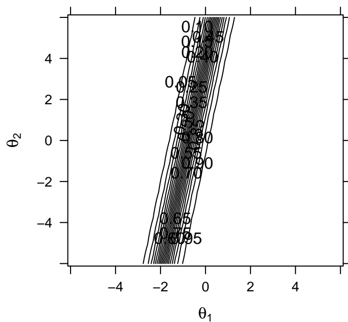
Futenma (rotate = 'promax')
