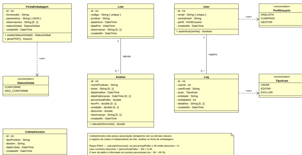
Diagrama de Classes — Modelo de Domínio do SCQ
