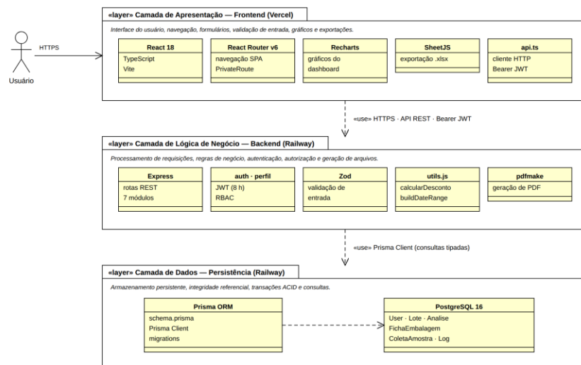
Diagrama de Pacotes — Arquitetura Cliente-Servidor em Três Camadas
