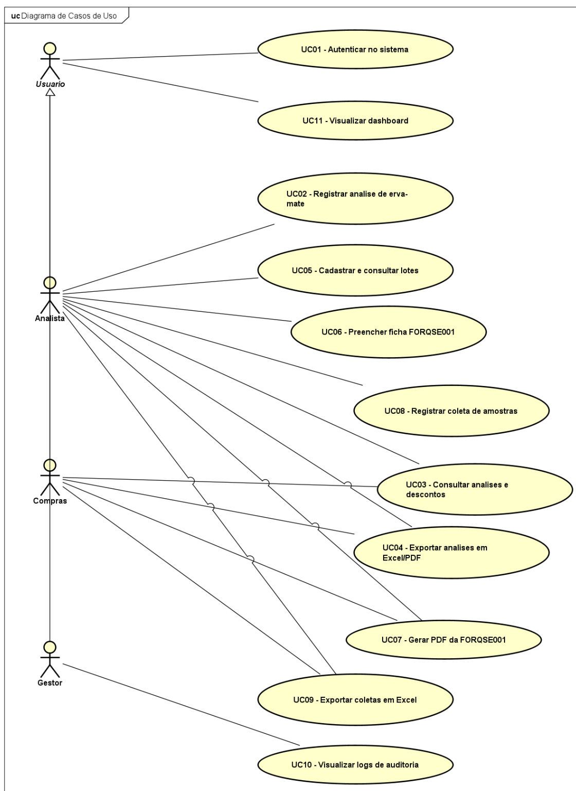
Figura 1 — Diagrama de casos de uso do SCQ.
