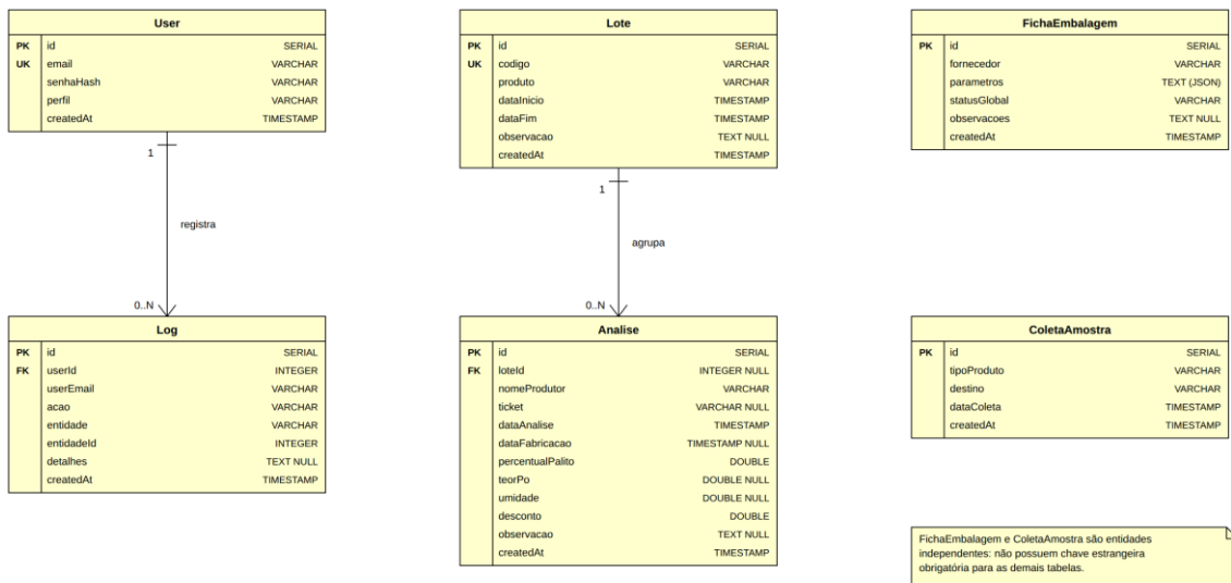
Figura 4 — Modelo entidade-relacionamento do banco de dados do SCQ.
