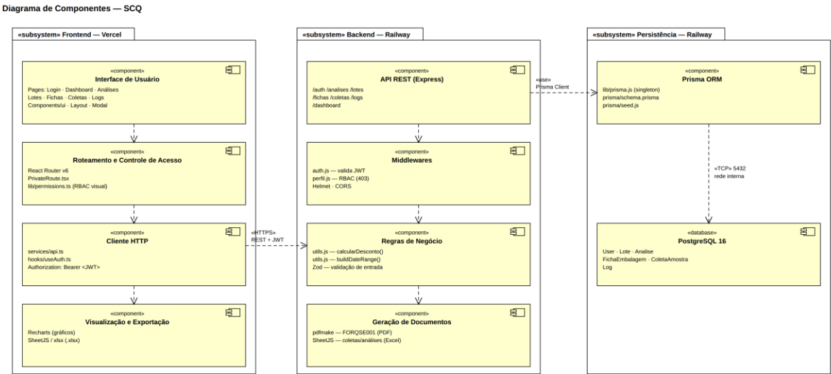
Figura 6 — Diagrama de componentes do SCQ.
