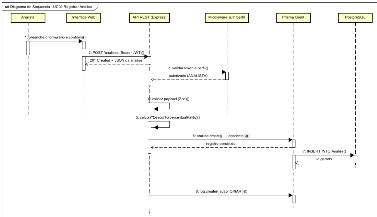
Figura 2 — Diagrama de sequência do caso de uso UC02 — registrar análise de erva-mate.
