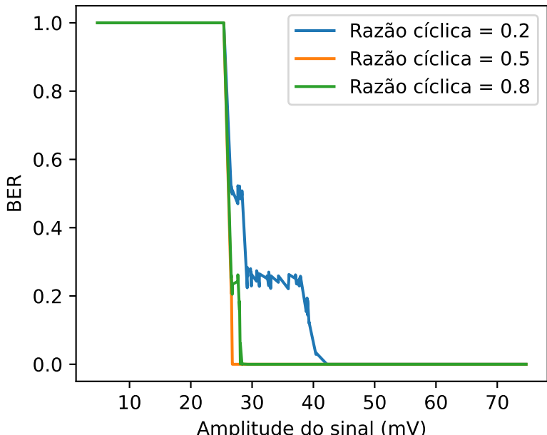
BER x Amplitude de V(compideal)_Trig
