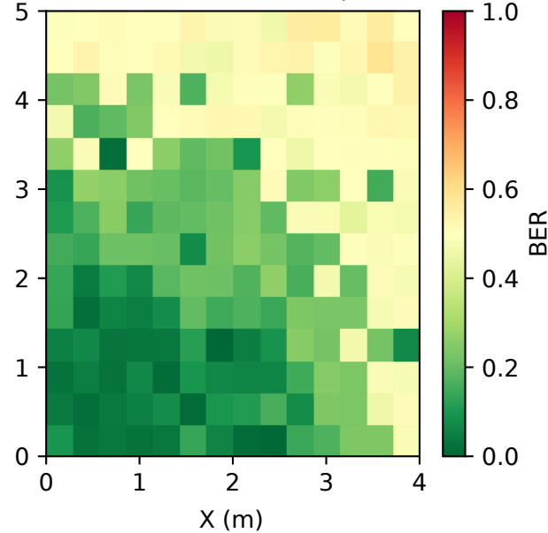
Razão cíclica = 0,8
