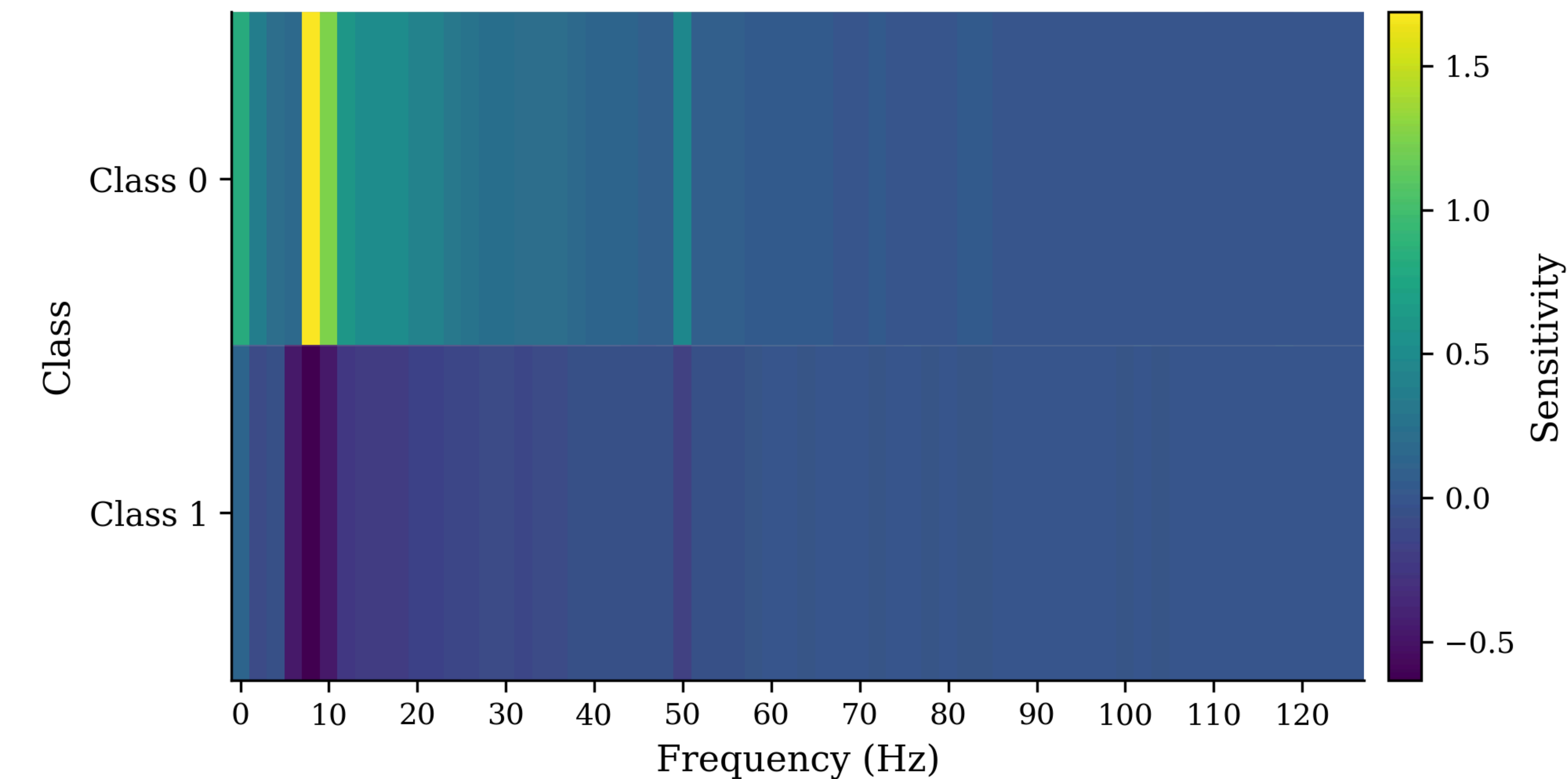
(a) APAVA Heatmap
