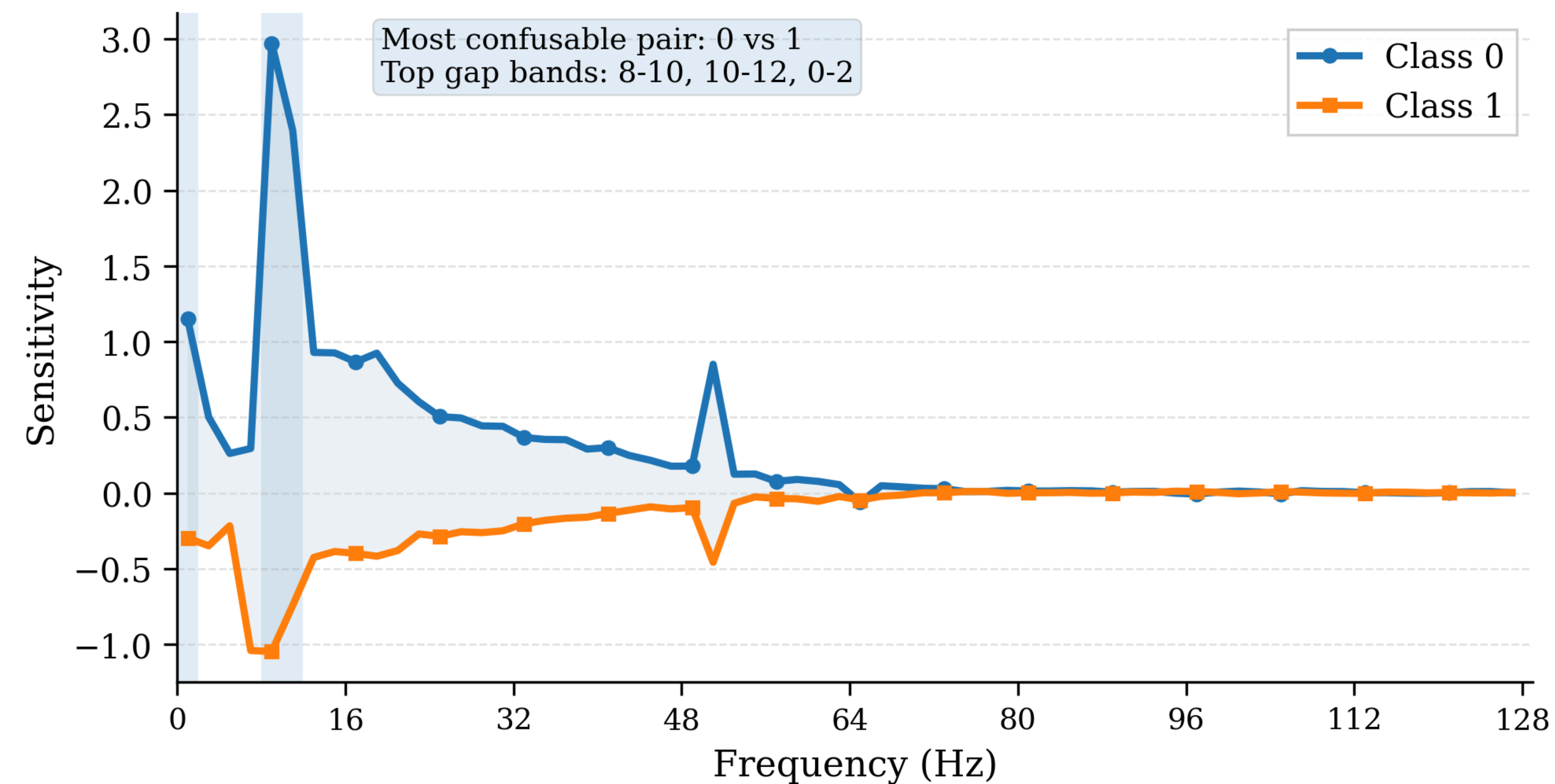
(b) APAVA w/o SCLN
