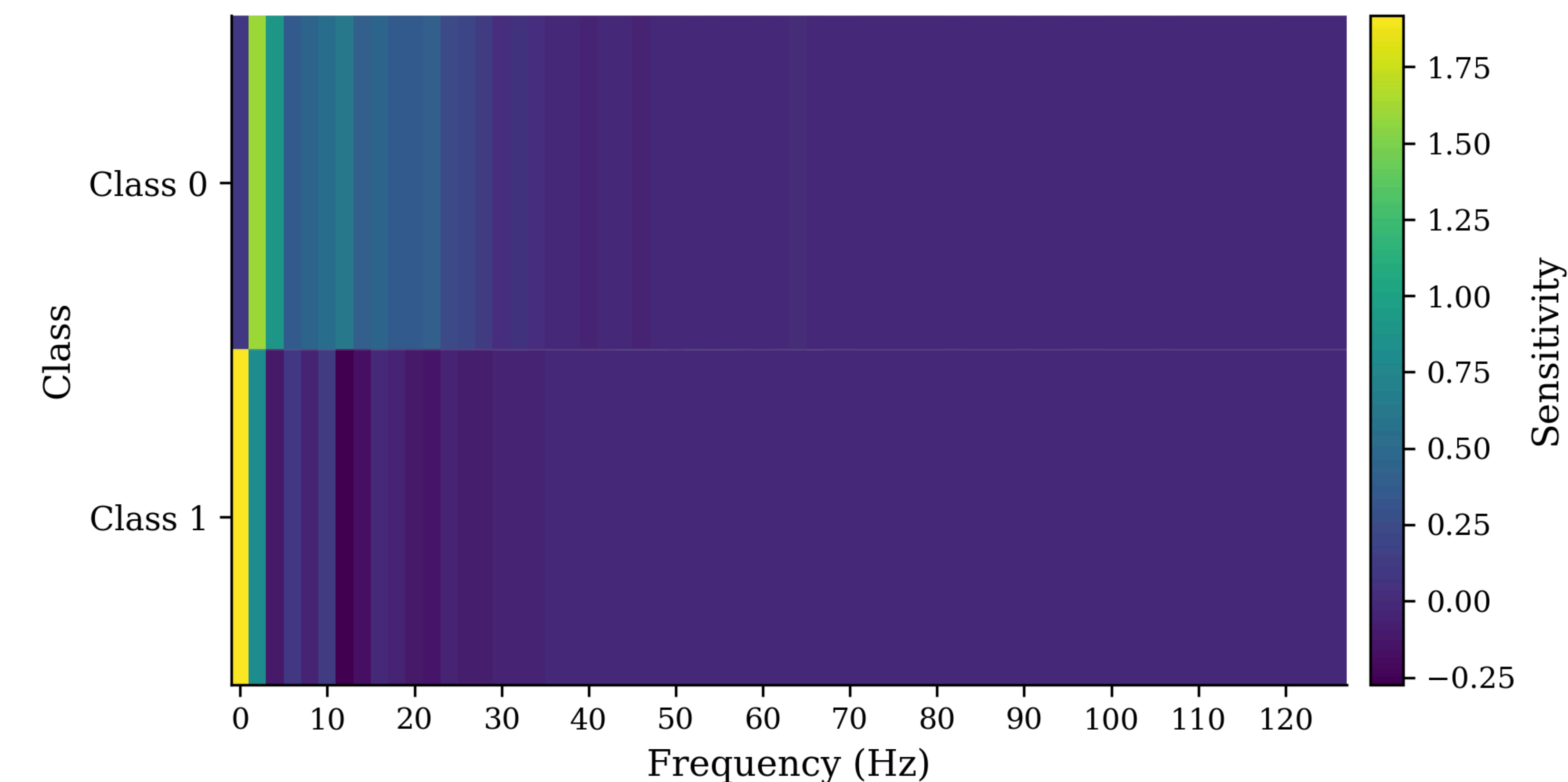
(d) PTB Heatmap
