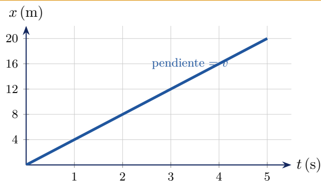
Figura 2.2: En el MRU, la gráfica posición–tiempo es una recta : su pendiente es la velocidad. Aquí v = 4 \text{ m/s} .
