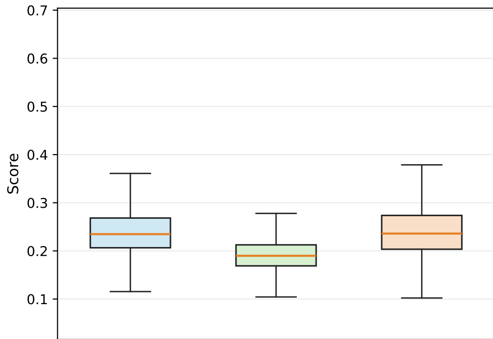
ROUGE-L F1
