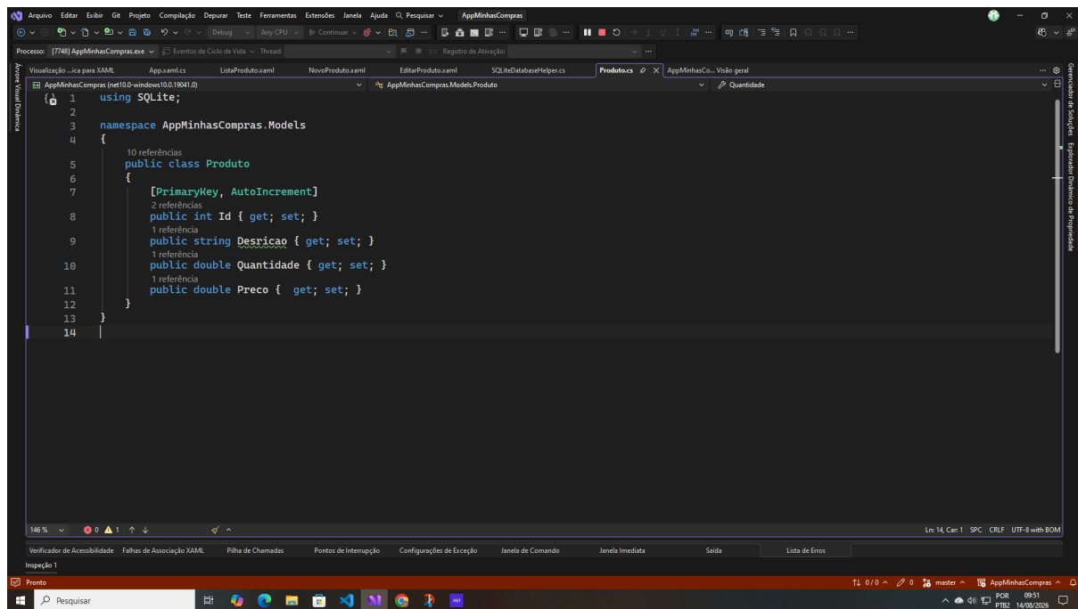
Imagem 6 - Classe Produto.cs
