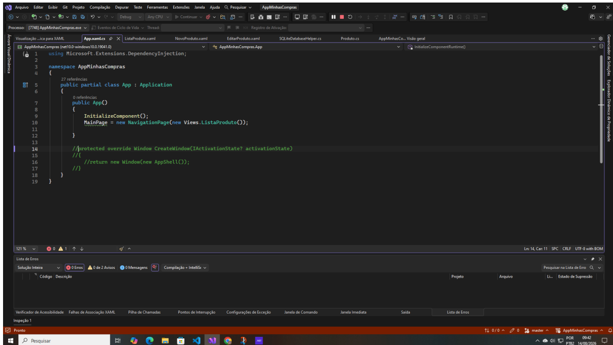
Imagem 1 - App.xaml.cs
