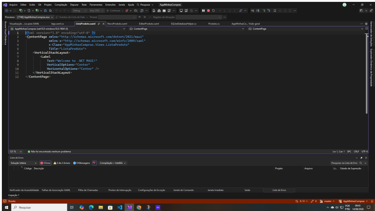
Imagem 2 - Item ListaProduto.xaml
