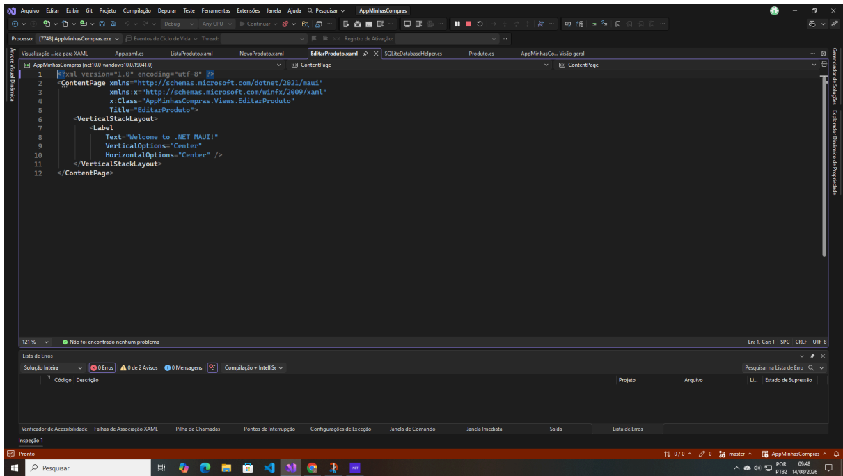
Imagem 4 - Item EditarProduto.xaml
