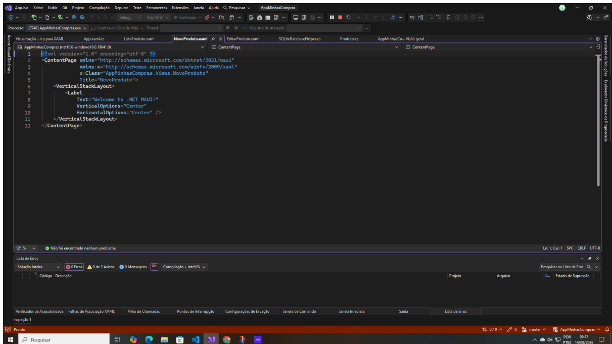
Imagem 3 - Item NovoProduto.xaml
