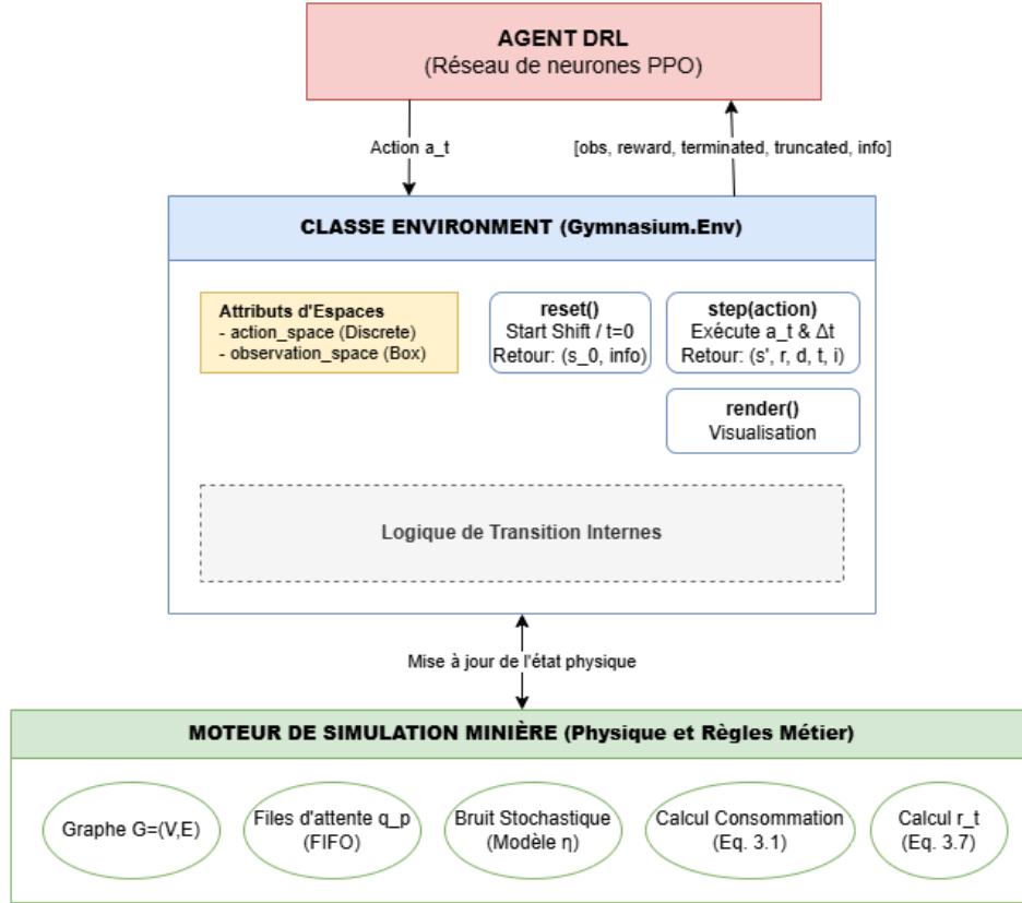
FIGURE 5.2 – Architecture modulaire de l'environnement MineEnv (Gymnasium).
