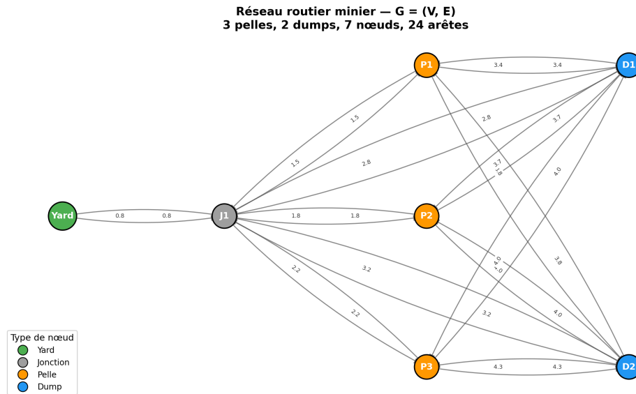
FIGURE 5.3 – Graphe routier du simulateur minier.
