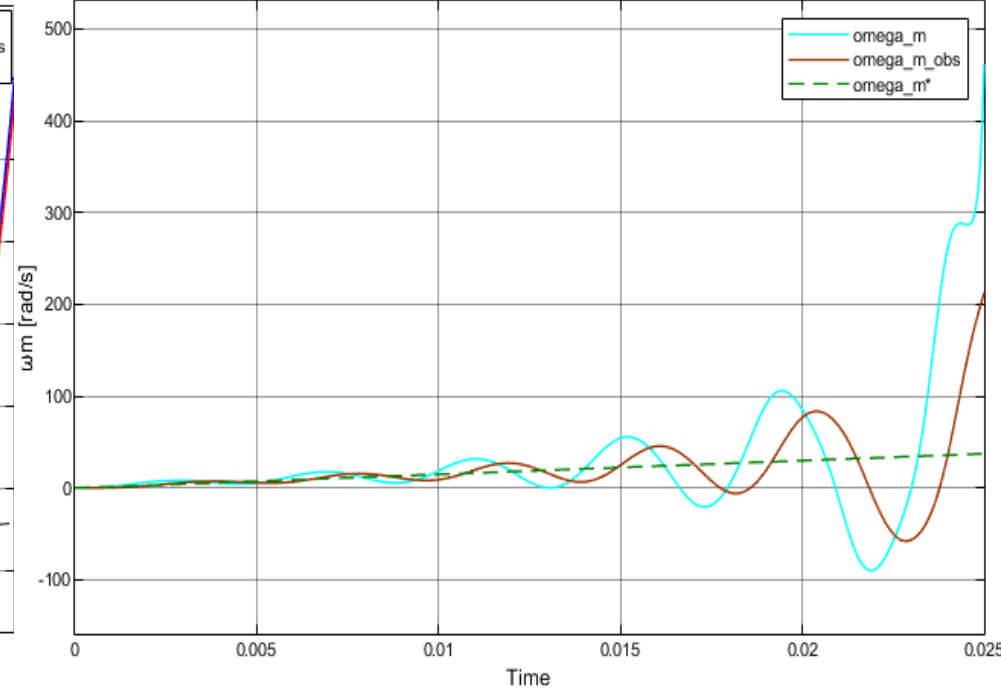
FIGURA: Figura 68— Curvas de velocidad con \omega_{n_{pos}} = 2000 \text{ rad/s}
