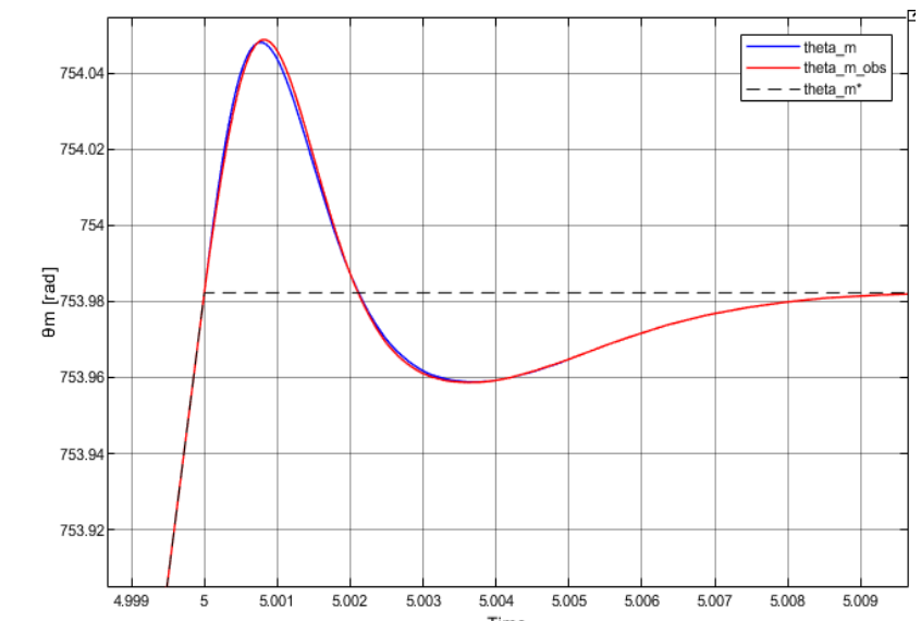
FIGURA: Figura 42— Figura 42: Detalle en t = 5s
