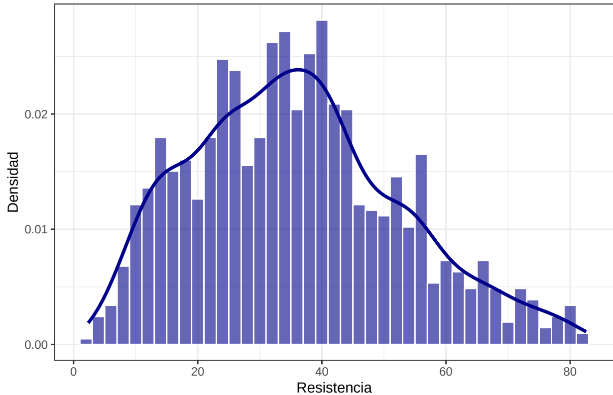
Distribución de la resistencia del concreto
