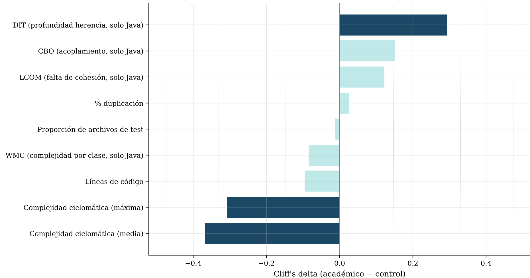
Fig. 4 — Tamaño del efecto por métrica (oscuro = significativo, Holm p < 0.05 )
