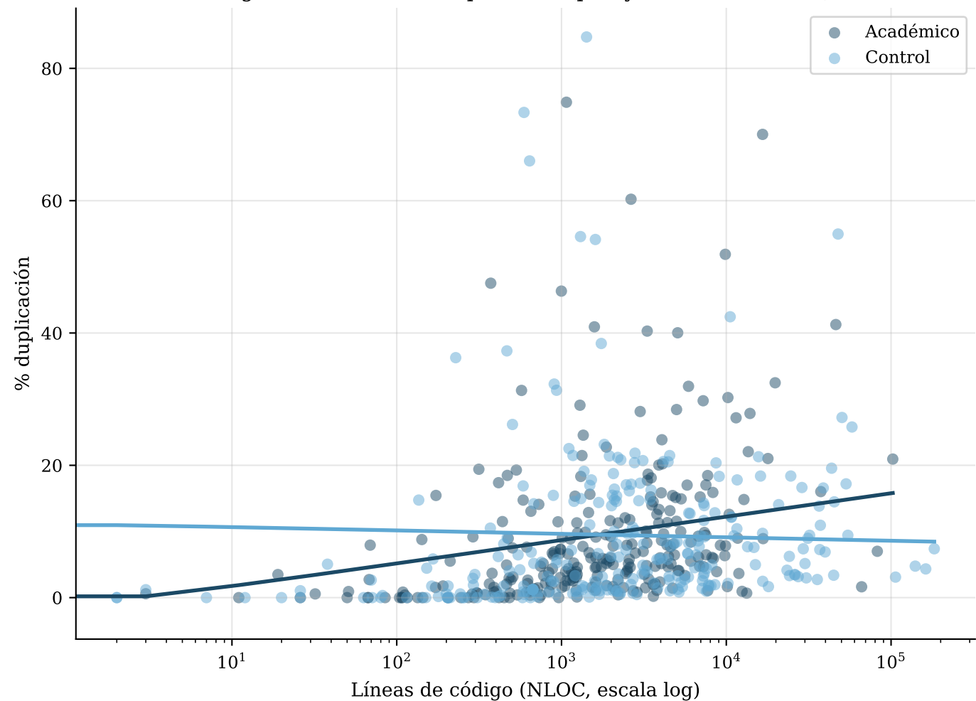
Fig. 3 — Tamaño vs. duplicación (proxy de deuda técnica)
