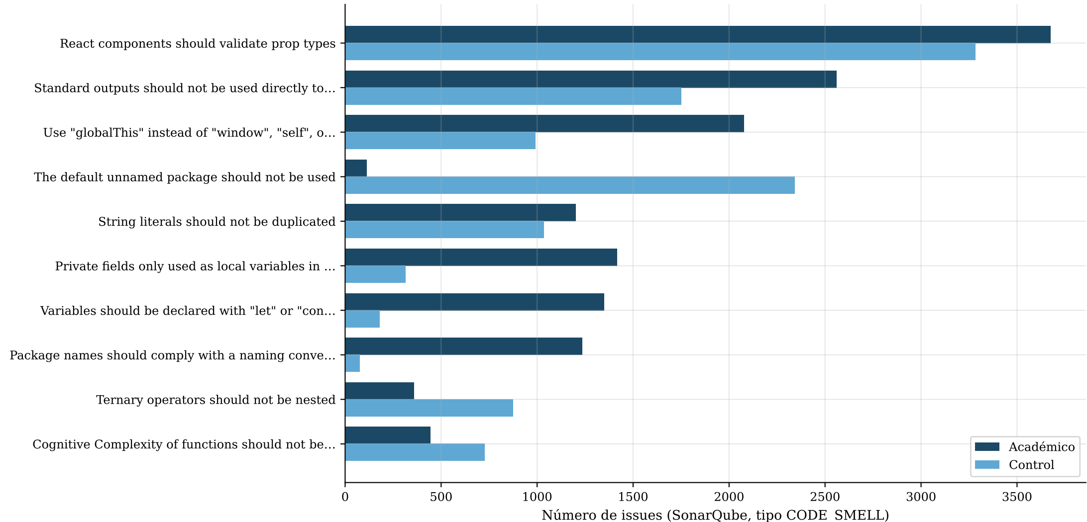
Fig. 4 — Los 10 tipos de code smell más frecuentes, académico vs. control (SonarQube Community, 415 repositorios analizados)
