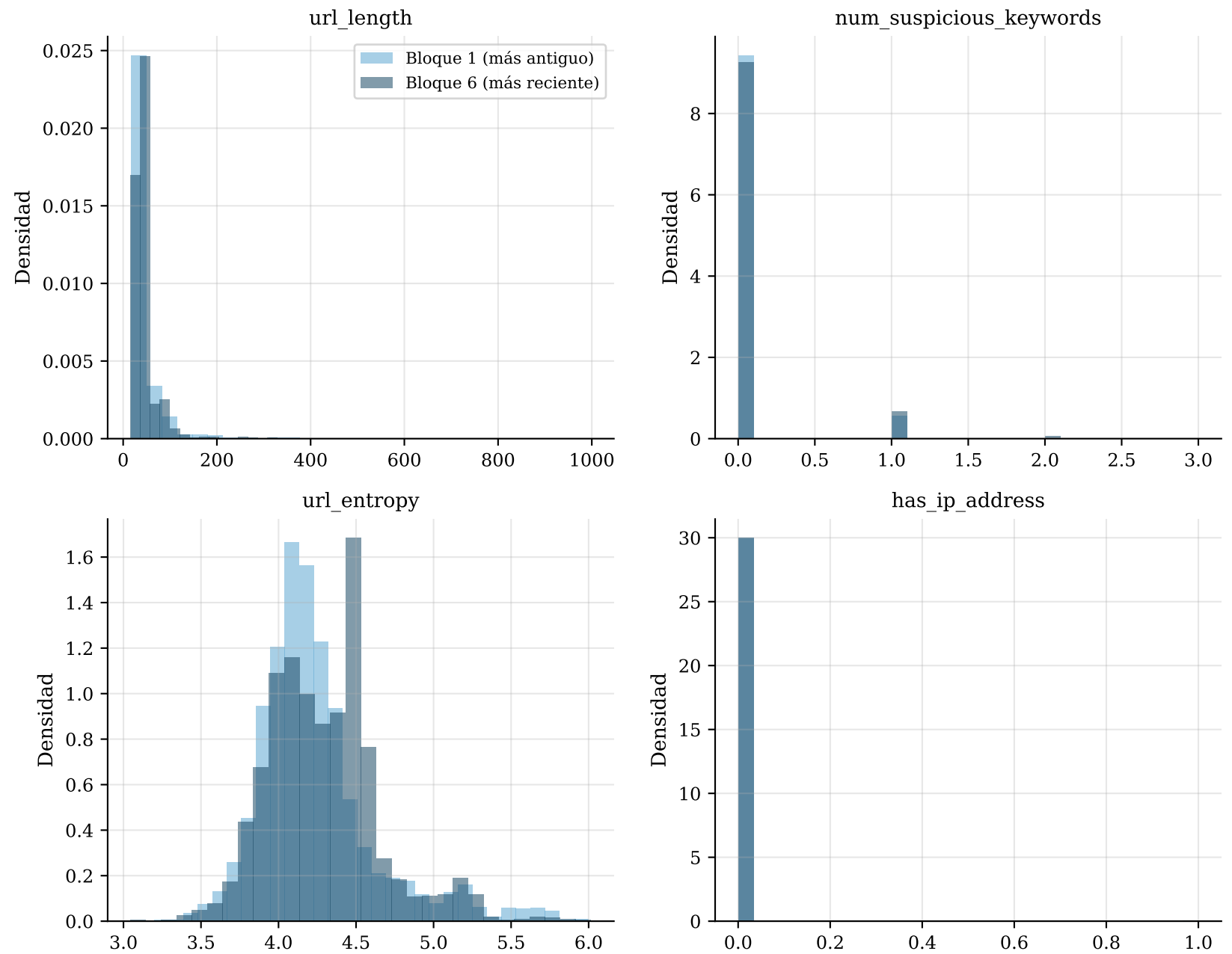
Fig. 3 — Desplazamiento de características clave (solo phishing) primer vs. último bloque temporal
