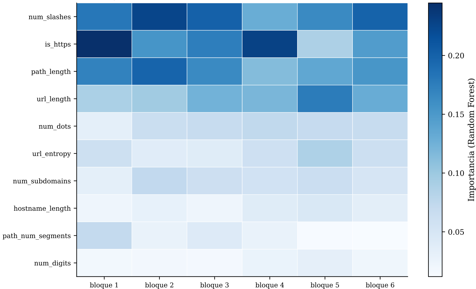
Fig. 4 — Importancia de características por bloque temporal
