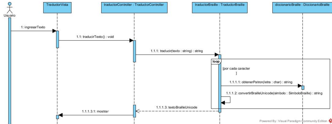
Figura 4. Diagrama secuencia CU01
