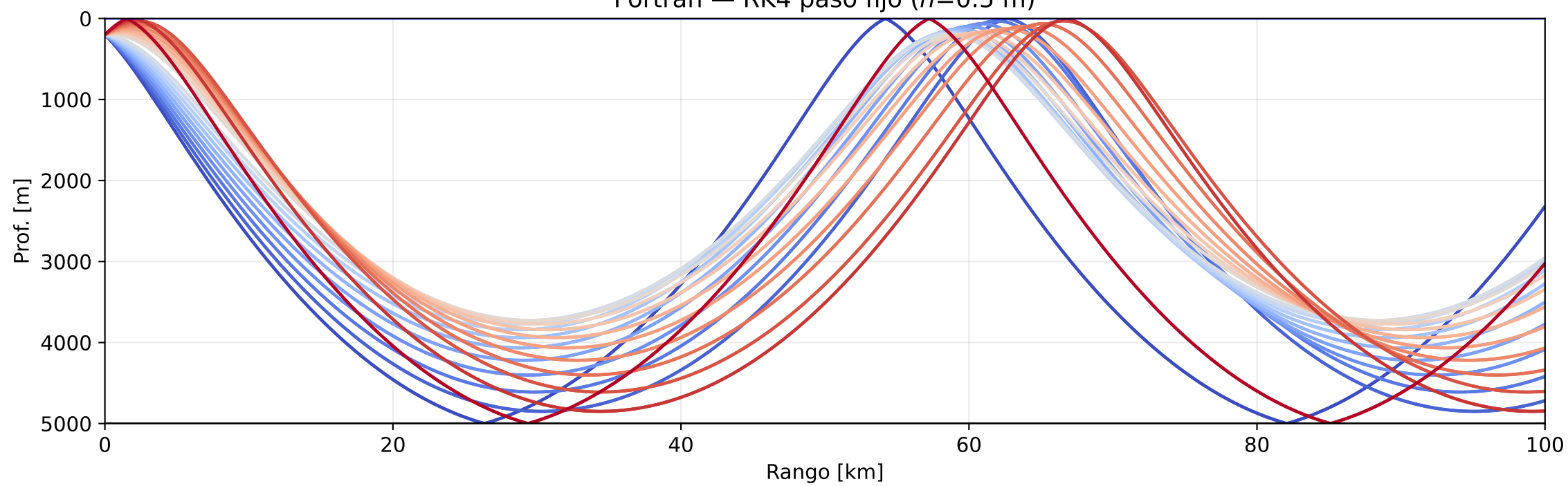
Fortran — RK4 paso fijo ( h=0.5 m)
