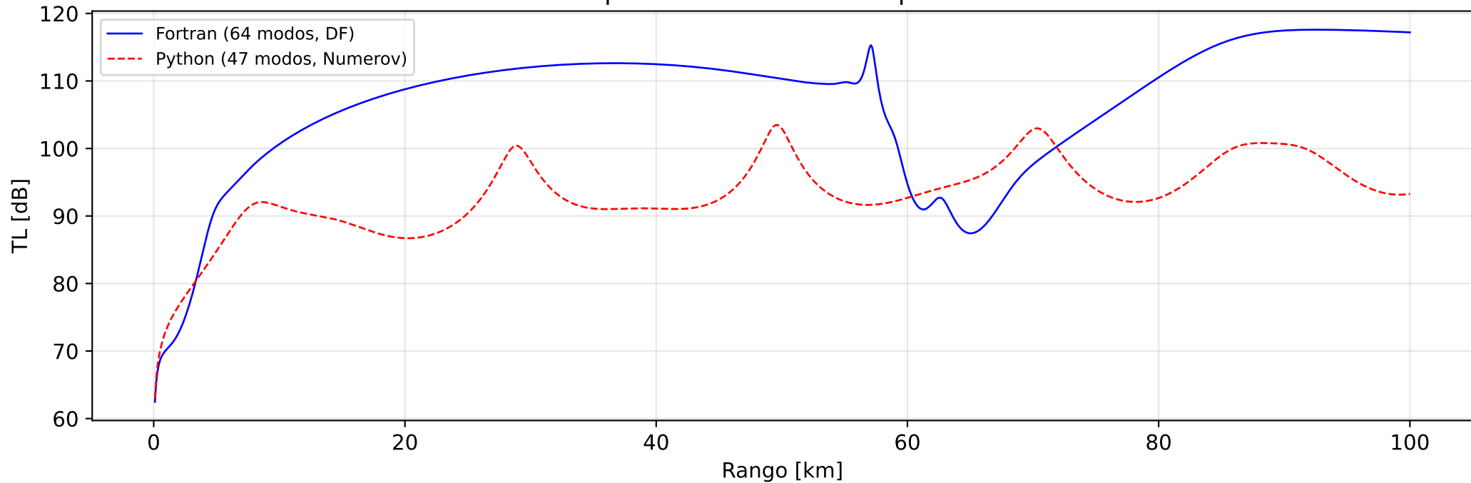
Pérdida por transmisión — receptor a 100 m
