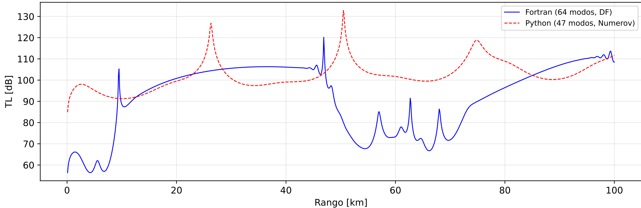
Pérdida por transmisión — receptor a 1000 m
