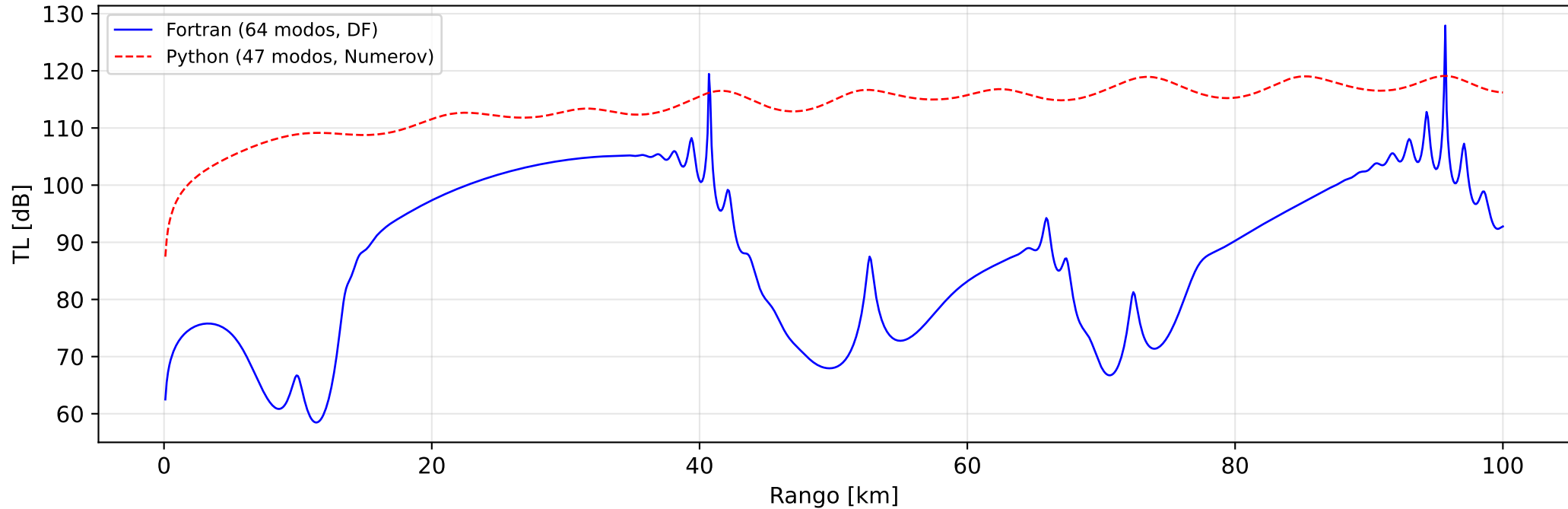
Pérdida por transmisión — receptor a 2000 m
